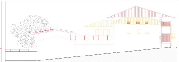
SOVRAPPOSIZIONE STATO DI FATTO-PROGETTO Prospetto sud - est
