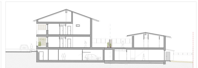
STATO DI FATTO Sezione A-A'
