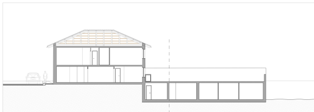
PROGETTO Sezione A-A'
