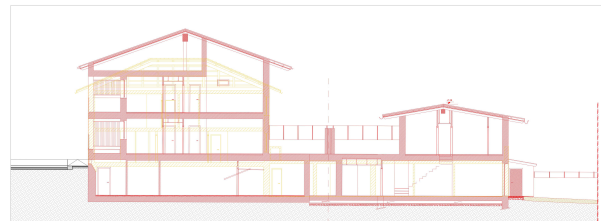
SOVRAPPOSIZIONE STATO DI FATTO-PROGETTO Sezione A-A'
