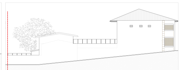
PROGETTO Prospetto sud - est
