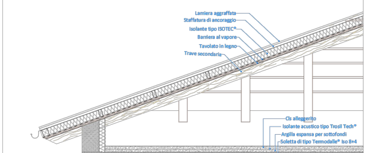
C Tipologia C: fanghiale continuo su piano primo
