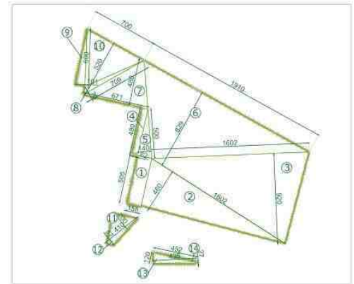
Estratto dell'elaborato "ED 5.8 Schema Planimetrico"
