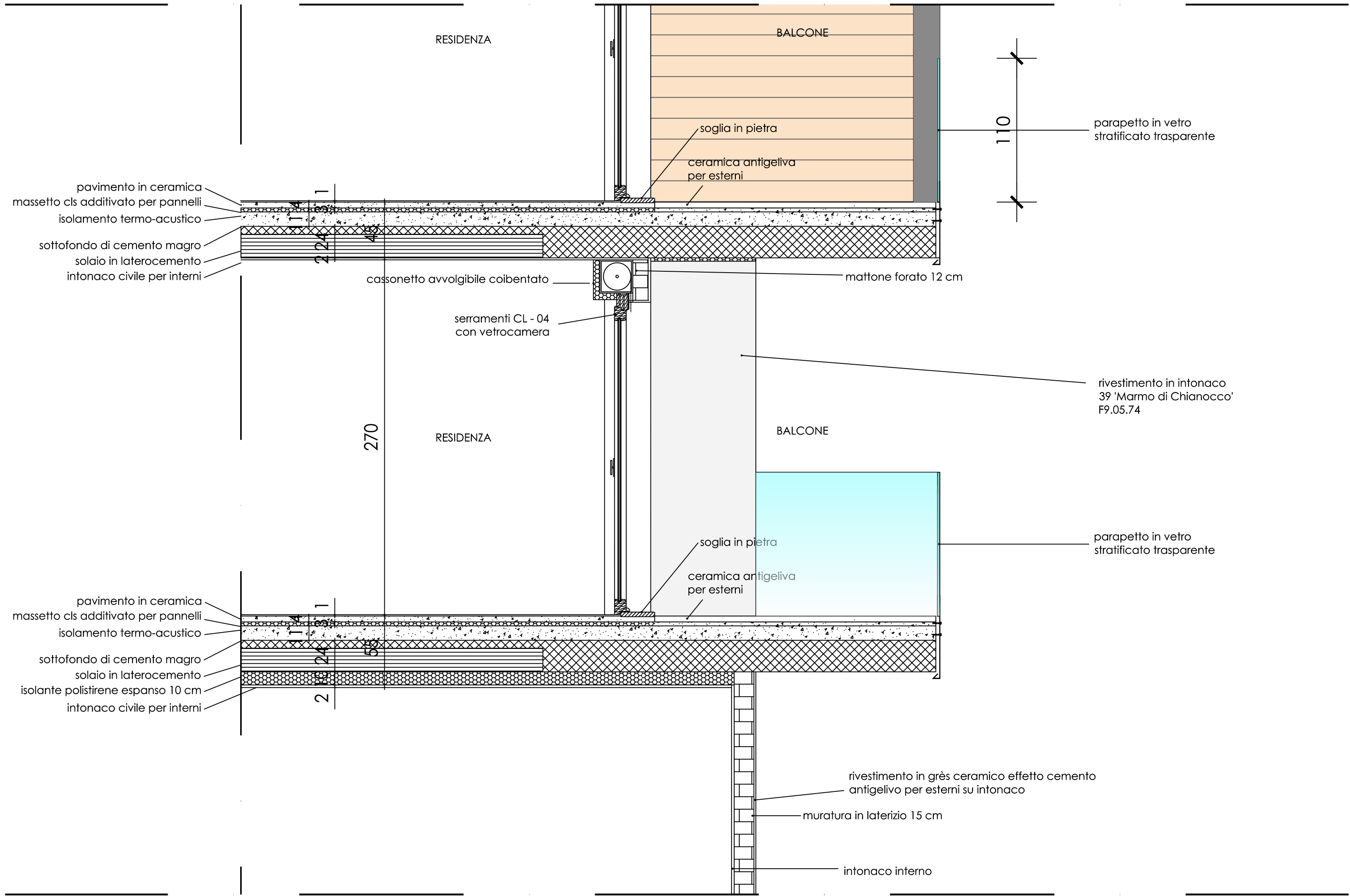
PARTICOLARE COSTRUTTIVO - SEZIONE 1:25
