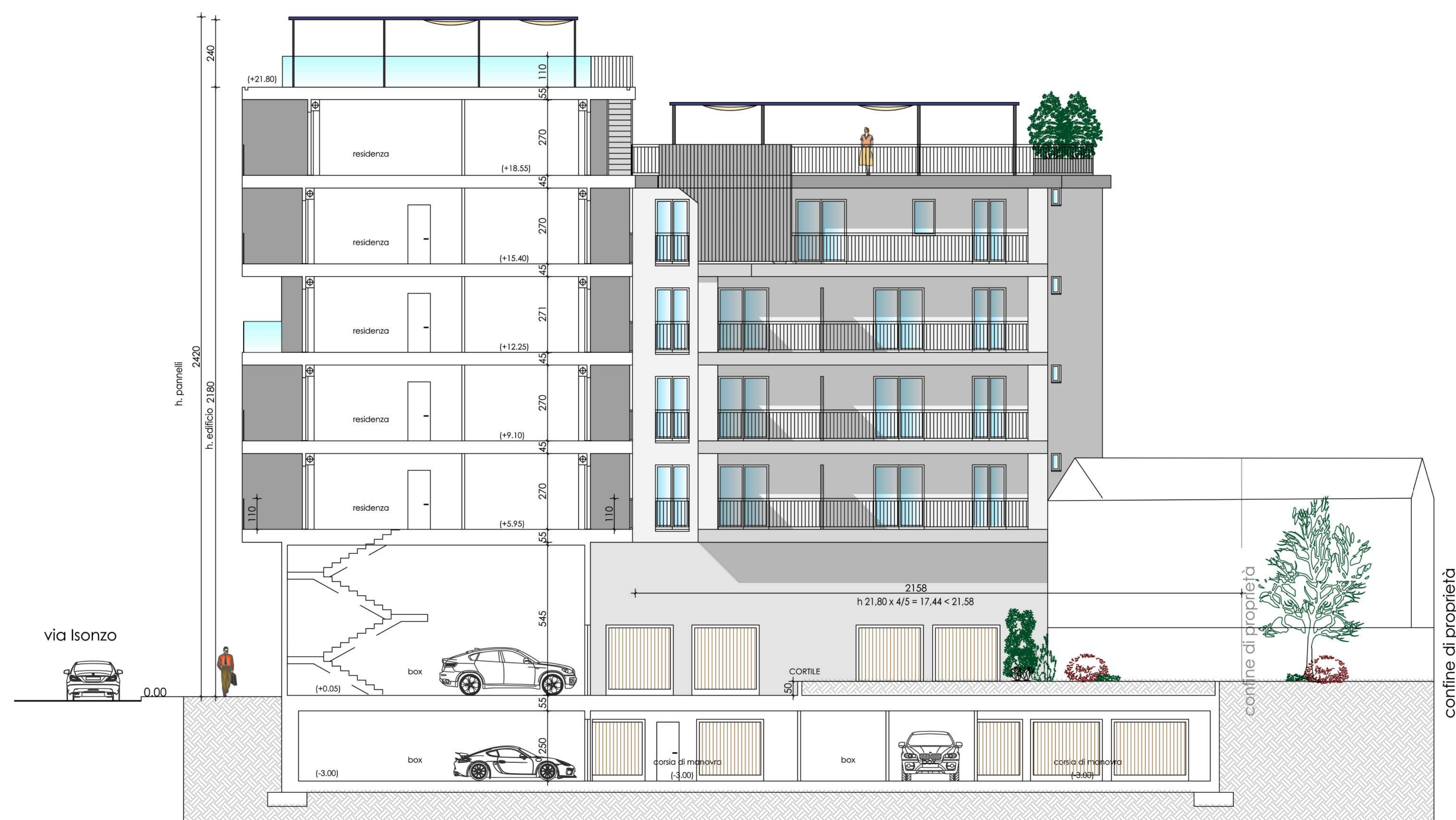
SEZIONE BB'
