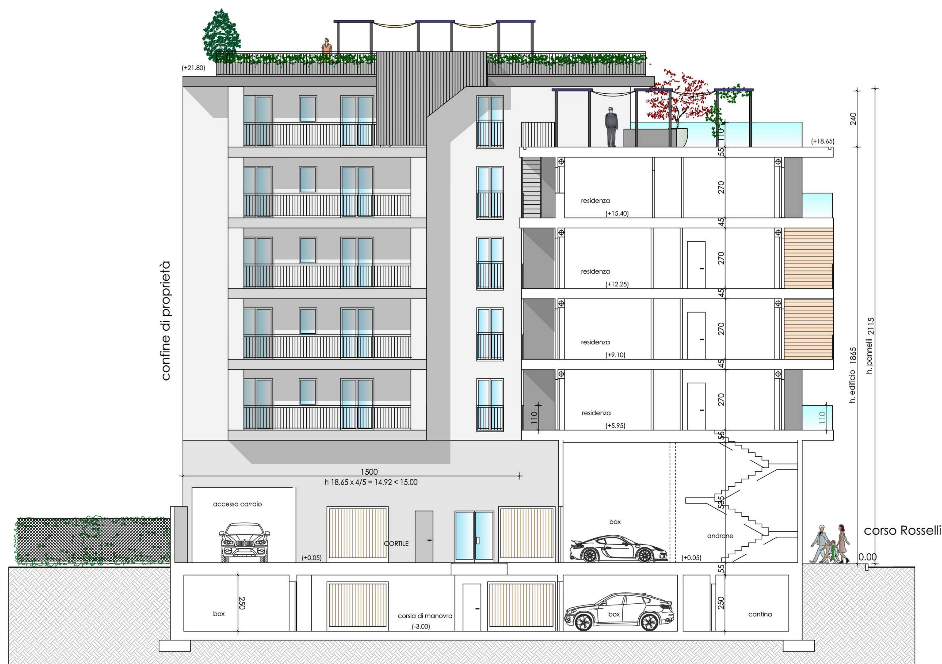
SEZIONE AA'
