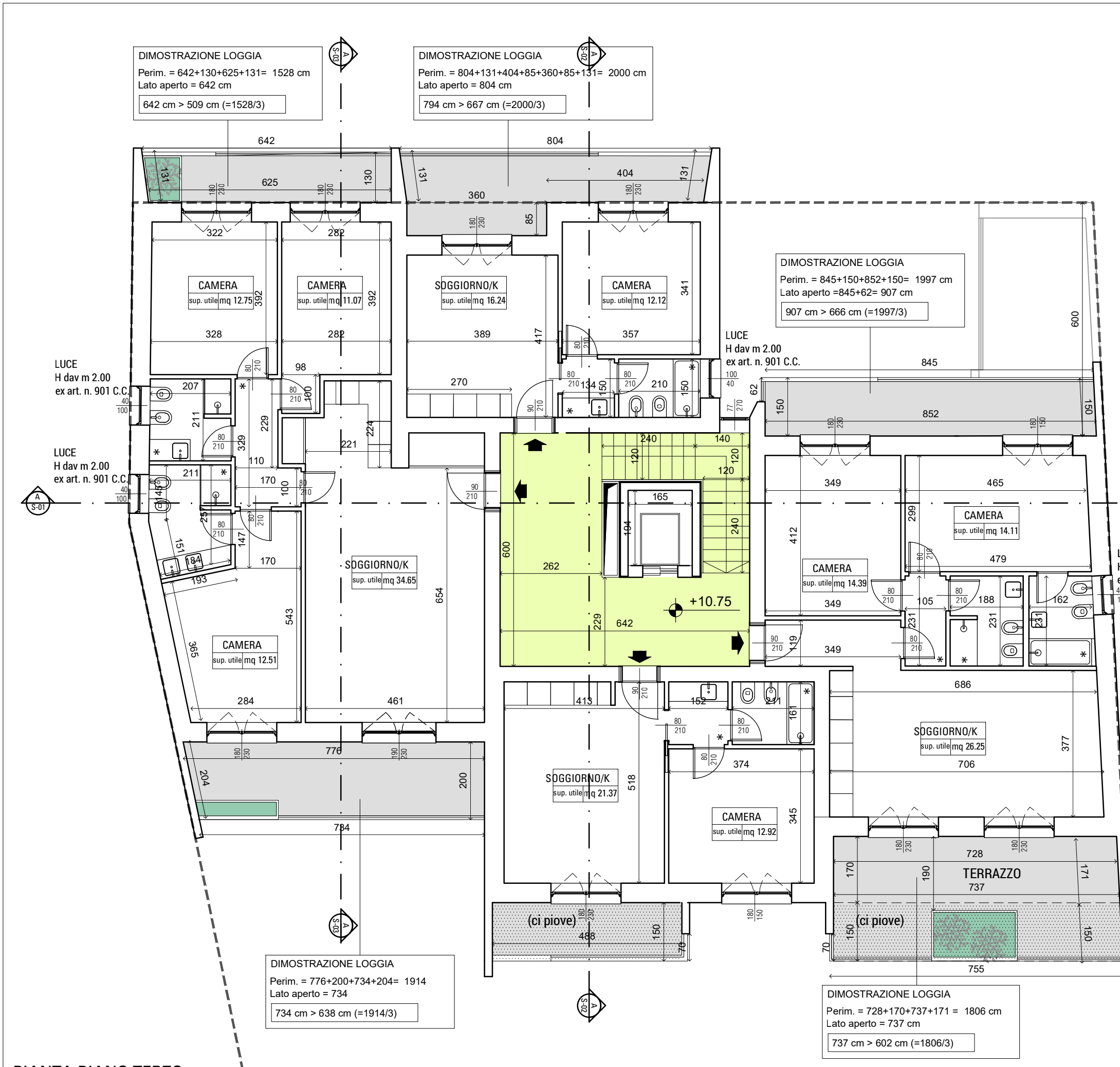
PIANTA PIANO TERZO
