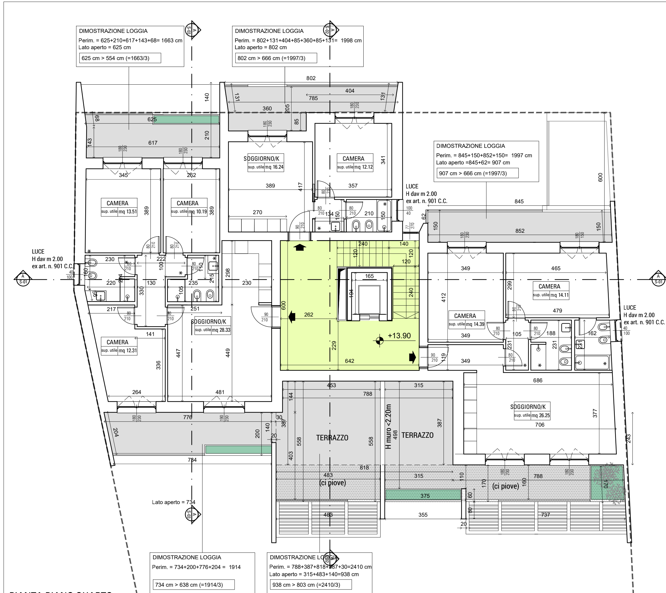
PIANTA PIANO QUARTO
