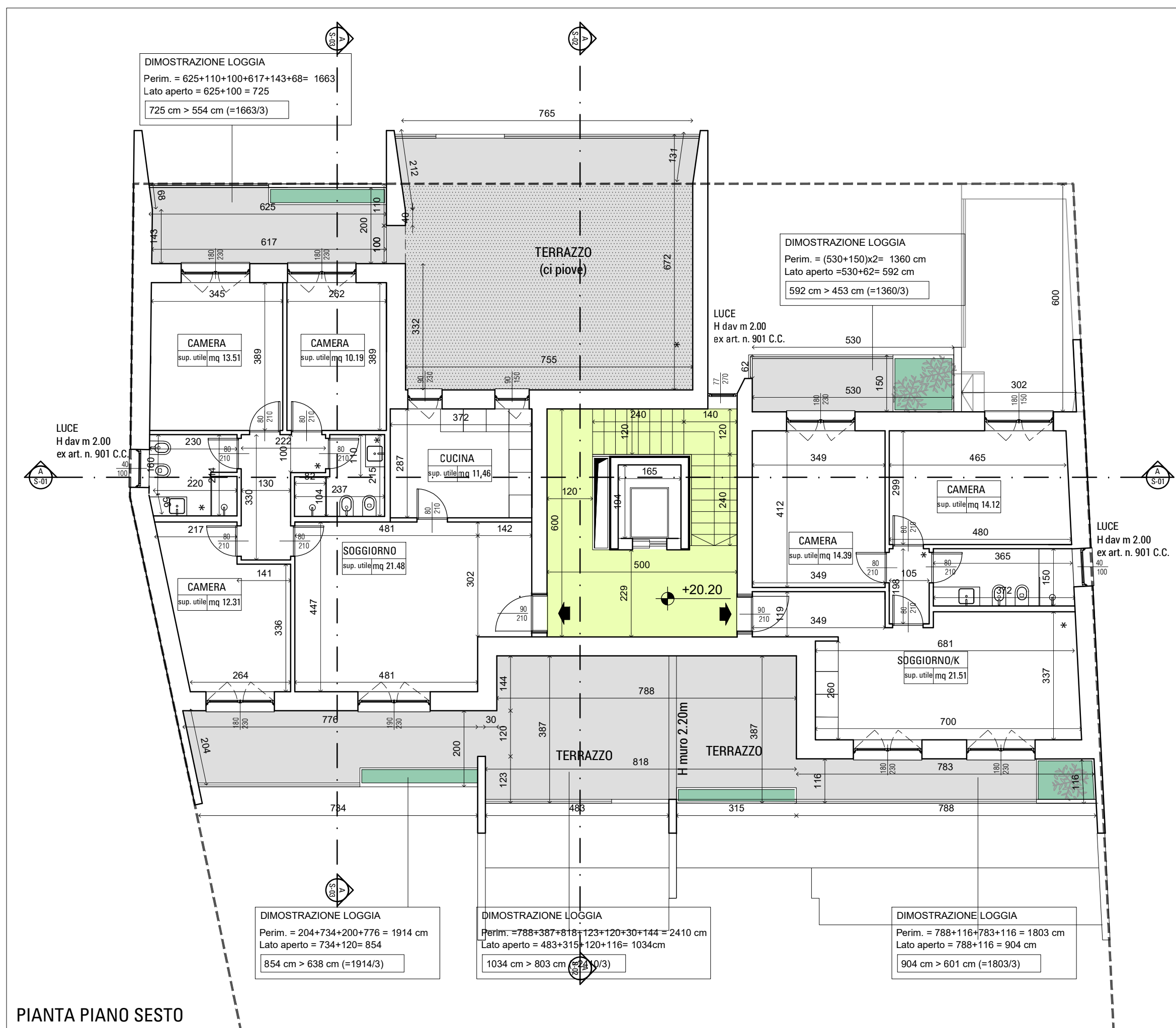
PIANTA PIANO SESTO
