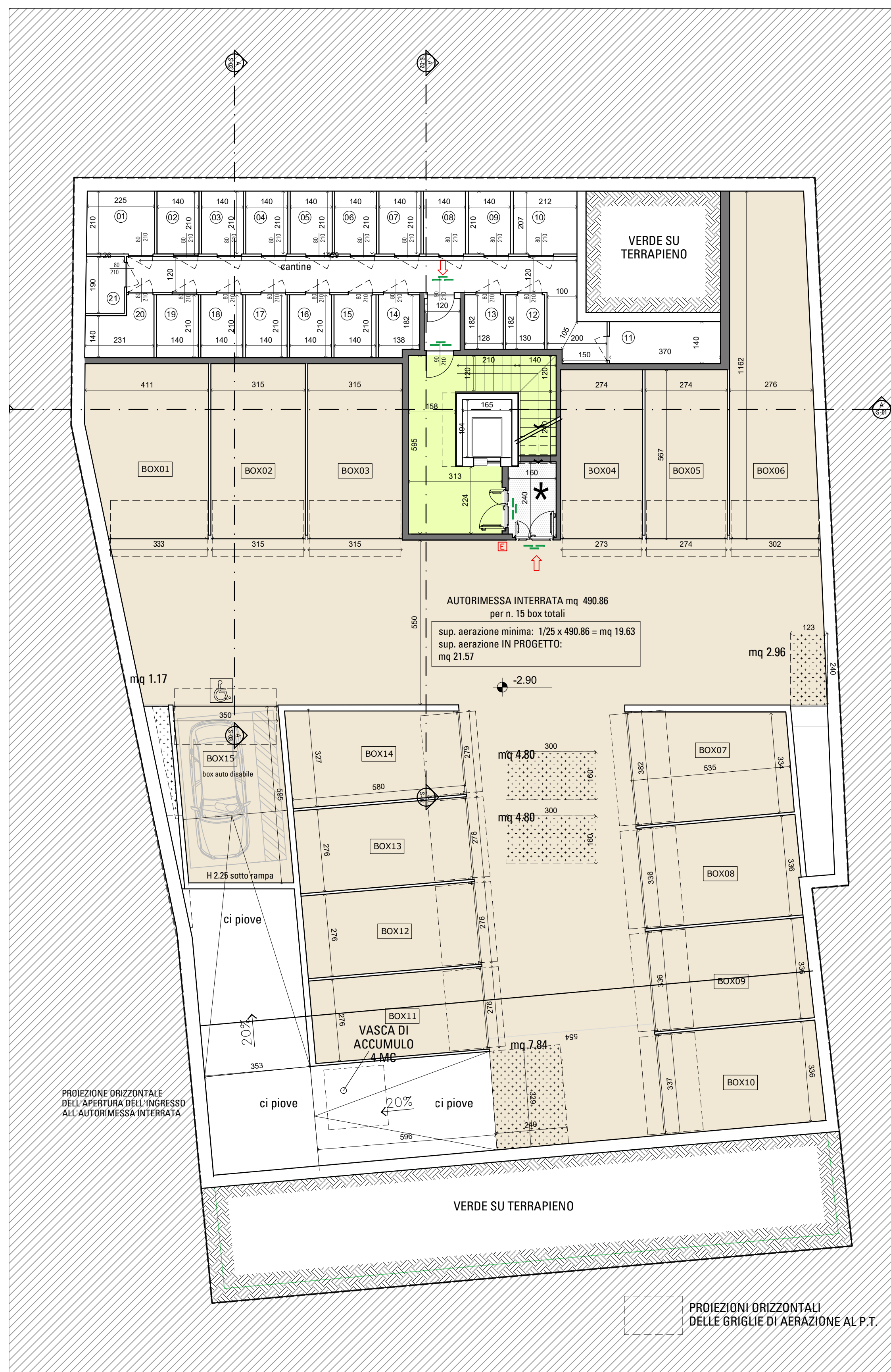
PIANTA PIANO INTERRATO
