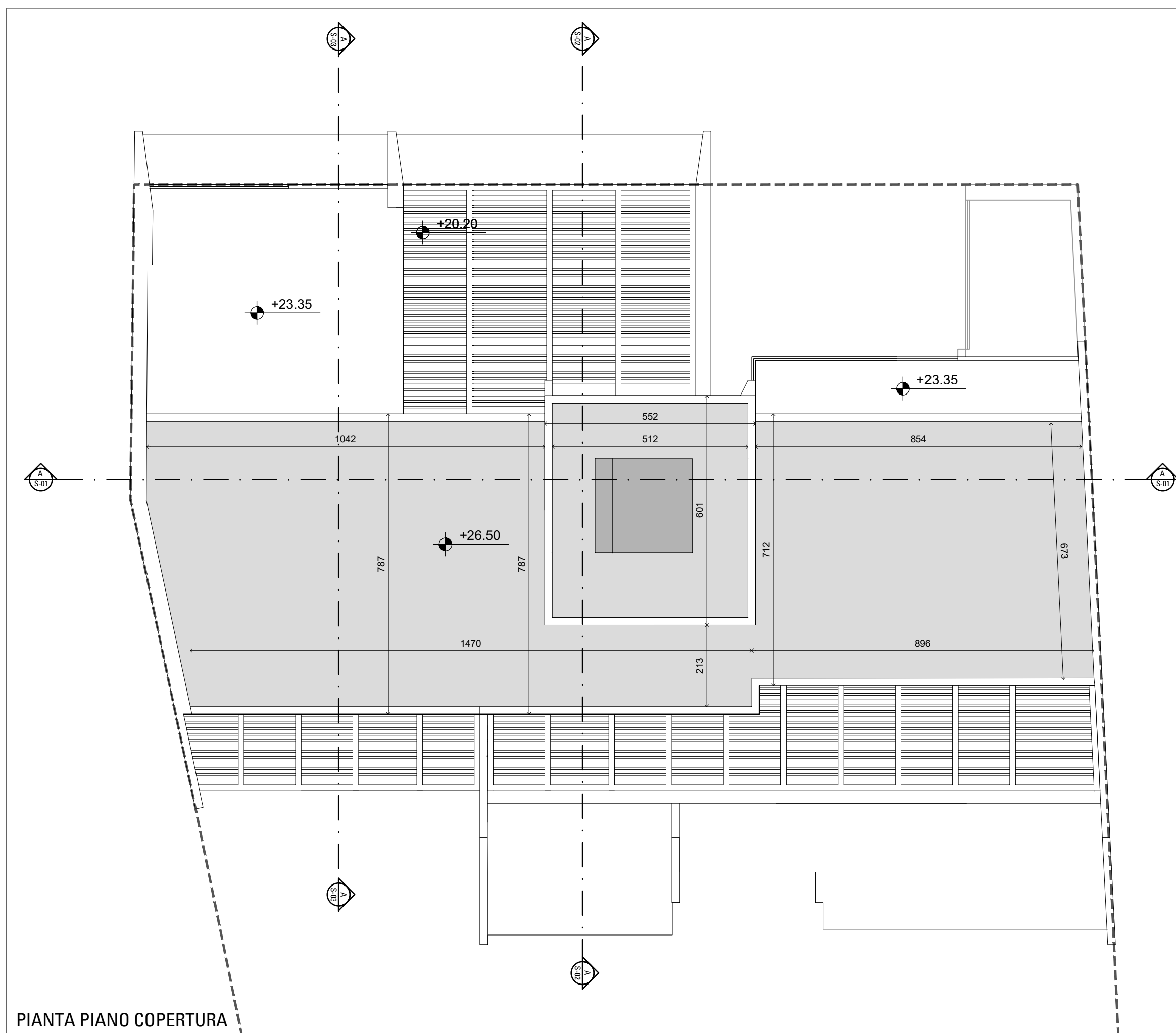
PIANTA PIANO COPERTURA
