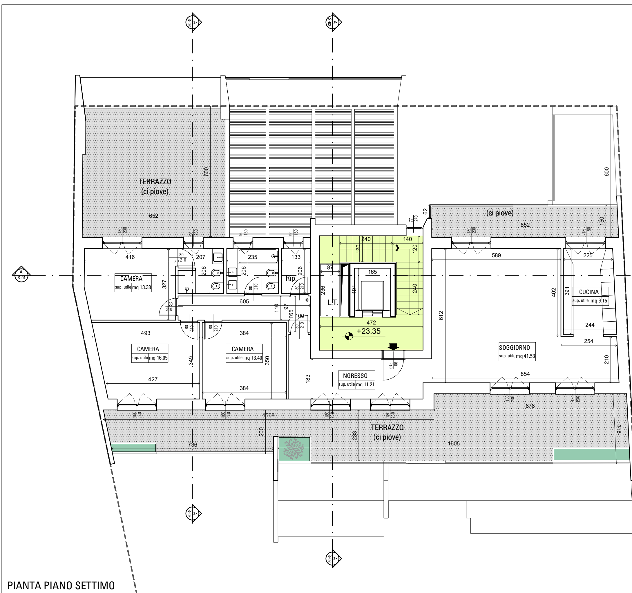
PIANTA PIANO SETTIMO
