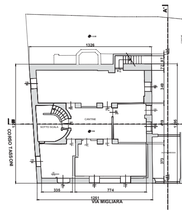
PIANTA PIANO SEMINTERRATO
