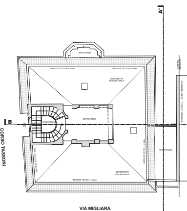
PIANTA PIANO SOTTOTETTO
