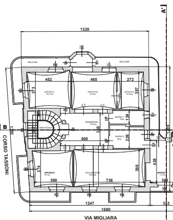
PIANTA PIANO PRIMO Foglio 1176 - Part. 368 - Sub. 5
