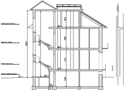
SEZIONE BB'
