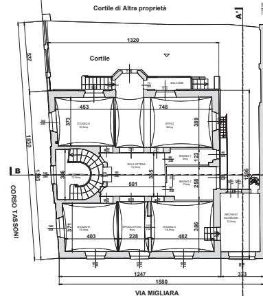
PIANTA PIANO TERRA RIALZATO Foglio 1176 - Part. 368 - Sub. 4
