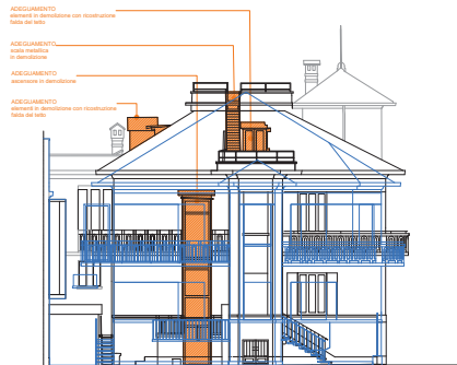
PROSPETTO NORD - Cortile nord
