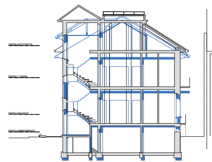
SEZIONE BB'
