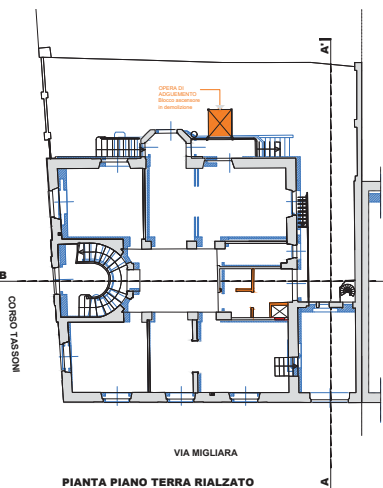
PIANTA PIANO TERRA RIALZATO Foglio 1176 - Part. 368 - Sub. 4
