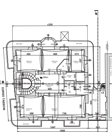
PIANTA PIANO PRIMO Foglio 1176 - Part. 368 - Sub. 5
