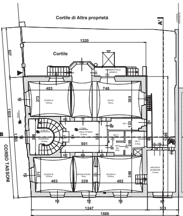
PIANTA PIANO TERRA RIALZATO Foglio 1176 - Part. 368 - Sub. 4
