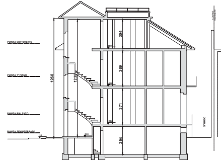
SEZIONE BB'
