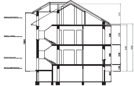
SEZIONE BB'
