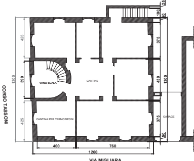
PIANTA PIANO SEMINTERRATO
