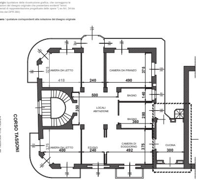
PIANTA PIANO PRIMO Foglio 1176 - Part. 368 - Sub. 5
