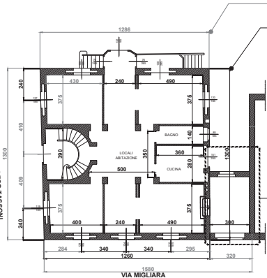
PIANTA PIANO TERRA RIALZATO Foglio 1176 - Part. 368 - Sub. 4
