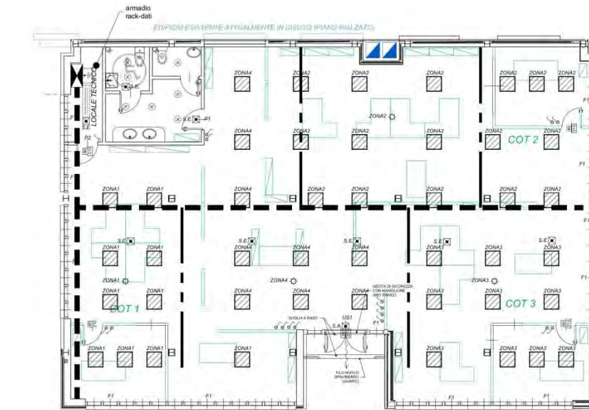
PLANIMETRIA IMPIANTO LUCE NORMALE/EMERGENZA-Scala 1:50
