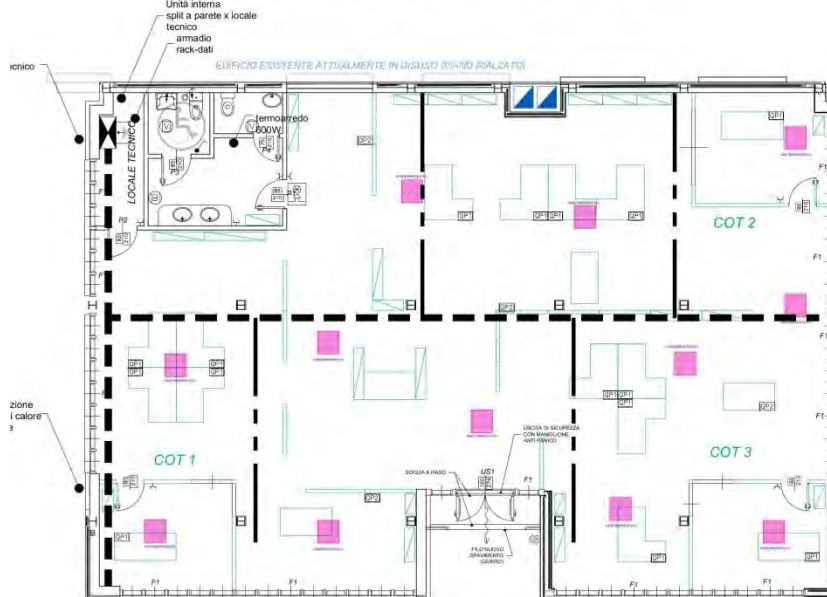
PLANIMETRIA IMPIANTO FORZA MOTRICE DI SERVIZIO-Scala 1:50
