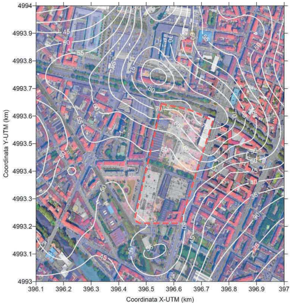
Figura 4-18: Scenario INT - Distribuzione spaziale delle concentrazioni medie annue di CO (valori in \mu\text{g}/\text{m}^3 )
