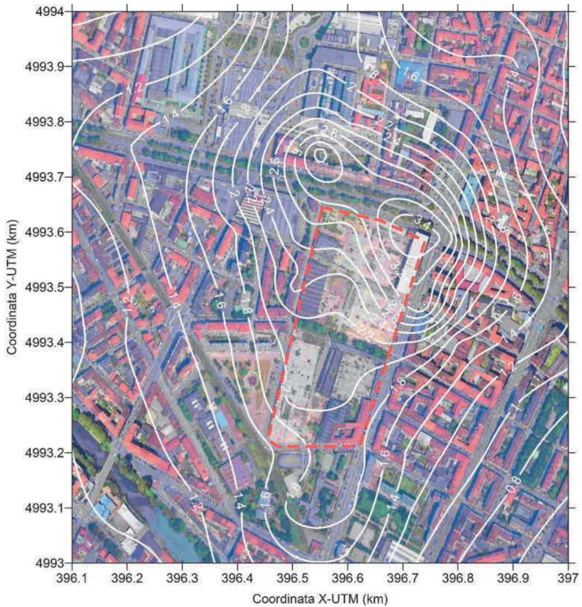
Figura 4-13: Scenario VARIANTE PRIN - Distribuzione spaziale delle concentrazioni medie annue di NO 2 (valori in µg/m 3 )
