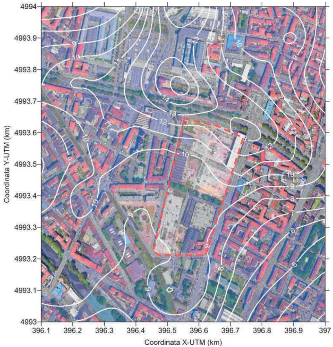
Figura 4-11: Scenario SDF - Distribuzione spaziale delle concentrazioni medie annue di NO 2 (valori in \mu\text{g}/\text{m}^3 )
