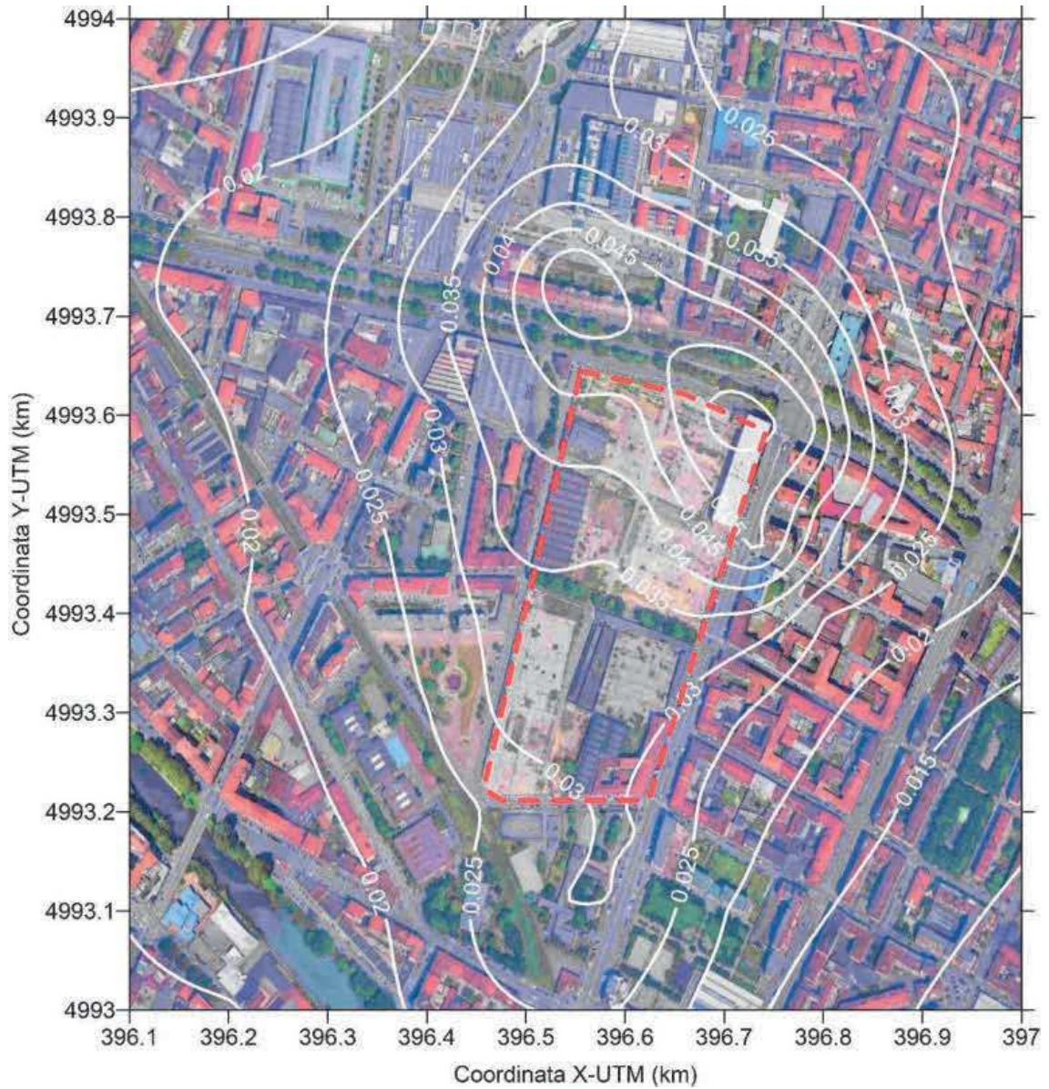
Figura 4-22: Scenario VARIANTE PRIN - Distribuzione spaziale delle concentrazioni medie annue di Benzene (valori in \mu\text{g}/\text{m}^3 )
