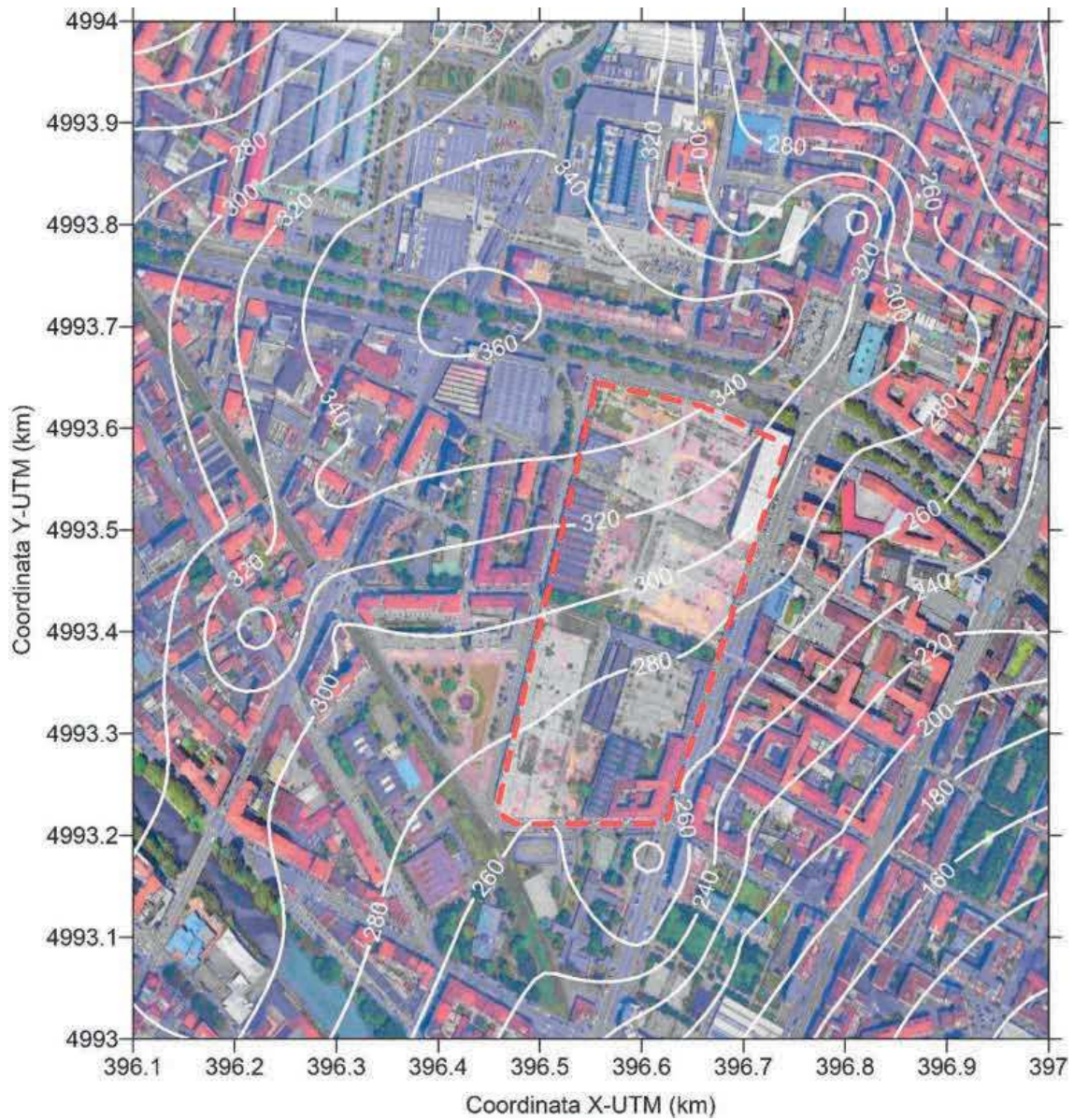
Figura 4-14: Scenario SDF - Distribuzione spaziale delle massime concentrazioni medie su 8 ore di CO (valori in \mu\text{g}/\text{m}^3 )
