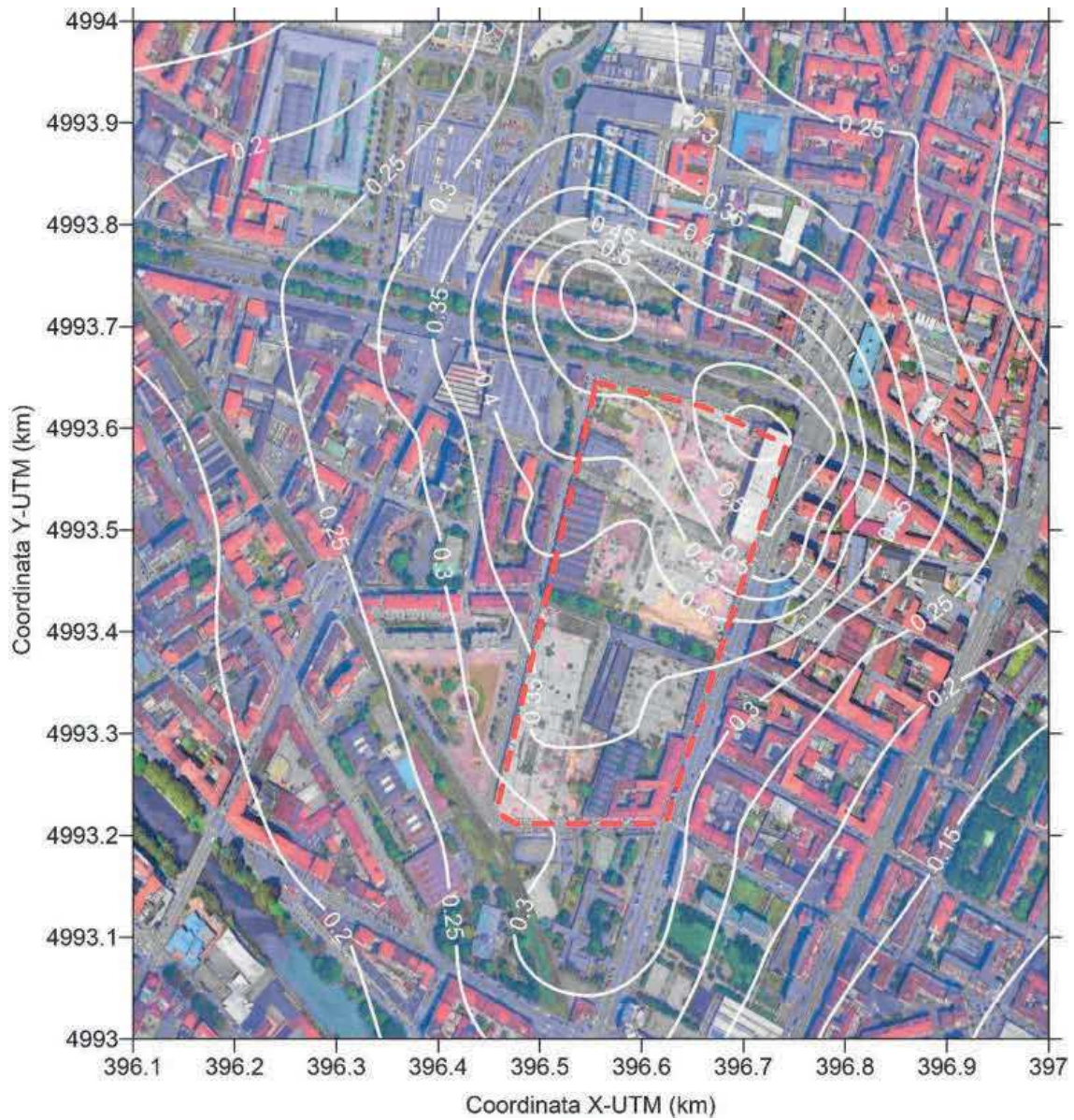
Figura 4-34: Scenario VARIANTE PRIN - Distribuzione spaziale delle concentrazioni medie annue di PM2.5 (valori in \mu\text{g}/\text{m}^3 )
