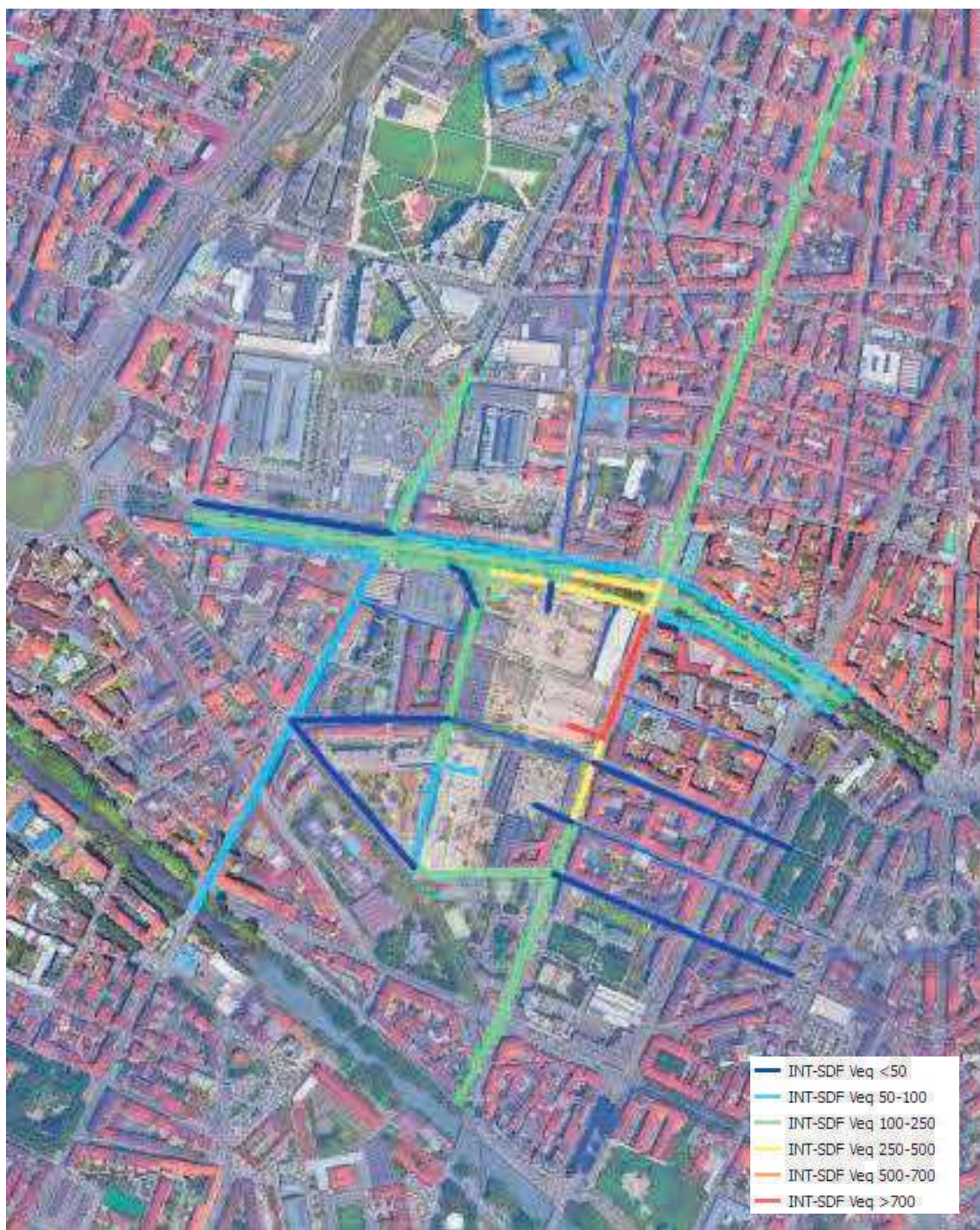
Figura 3-3 Scenario VARIANTE PRIN Veicoli equivalenti Ora di punta
