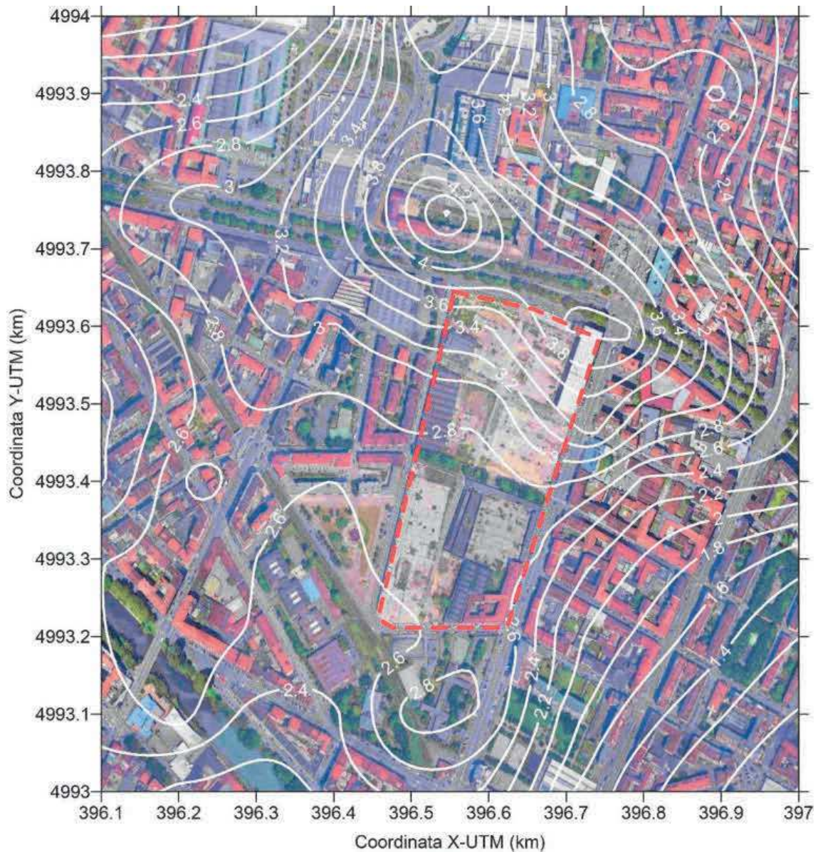
Figura 4-30: Scenario INT - Distribuzione spaziale delle concentrazioni medie annue di PM10 (valori in \mu\text{g}/\text{m}^3 )
