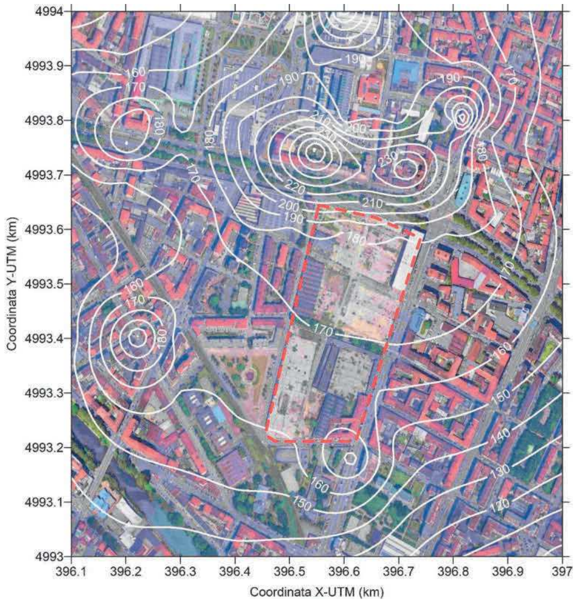
Figura 4-6: Scenario INT - Distribuzione spaziale delle concentrazioni massime orarie di NO 2 (valori in \mu\text{g}/\text{m}^3 )
