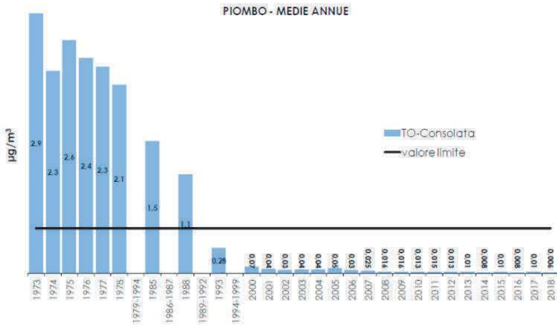
Figura 2-13 Piombo Concentrazione media annua
