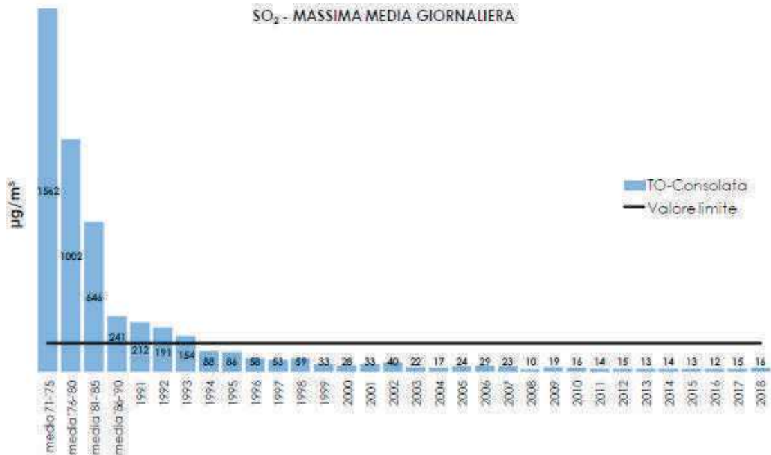
Figura 2-5 SO 2 Massima concentrazione media giornaliera
