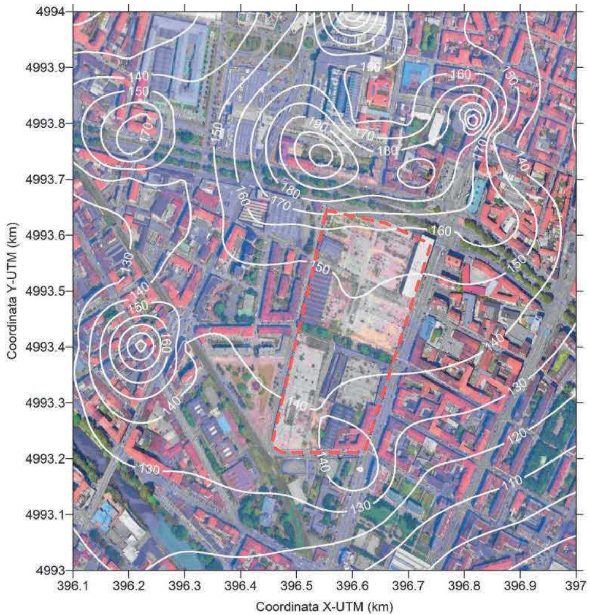
Figura 4-5: Scenario SDF - Distribuzione spaziale delle concentrazioni massime orarie di NO 2 (valori in µg/m 3 )
