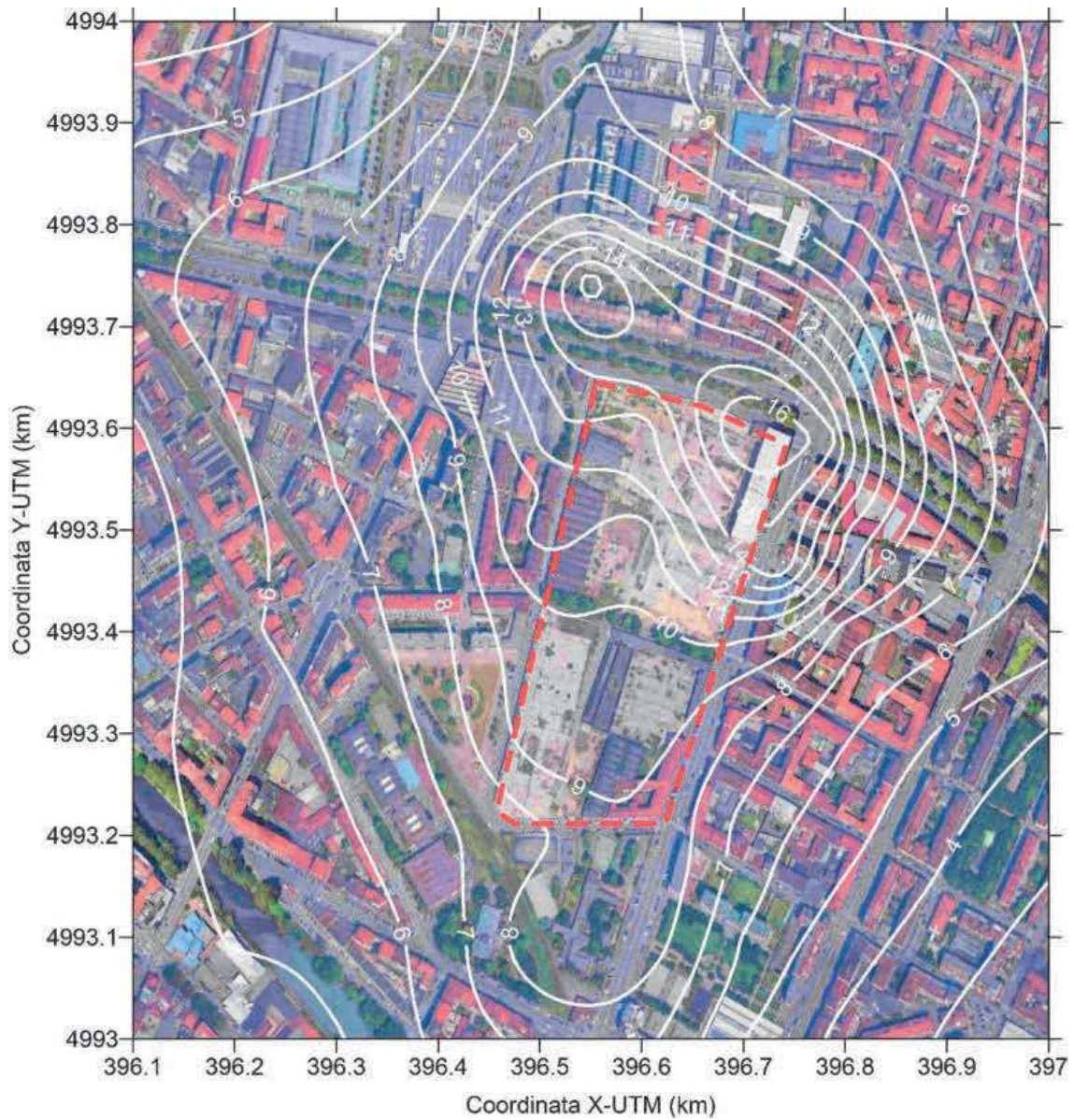
Figura 4-19: Scenario VARIANTE PRIN - Distribuzione spaziale delle concentrazioni medie annue di CO (valori in \mu\text{g}/\text{m}^3 )
