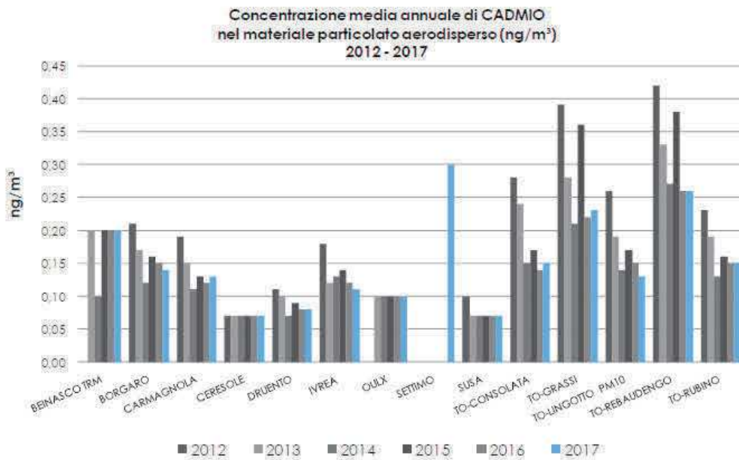
Figura 2-14 Cadmio Concentrazione media annua
