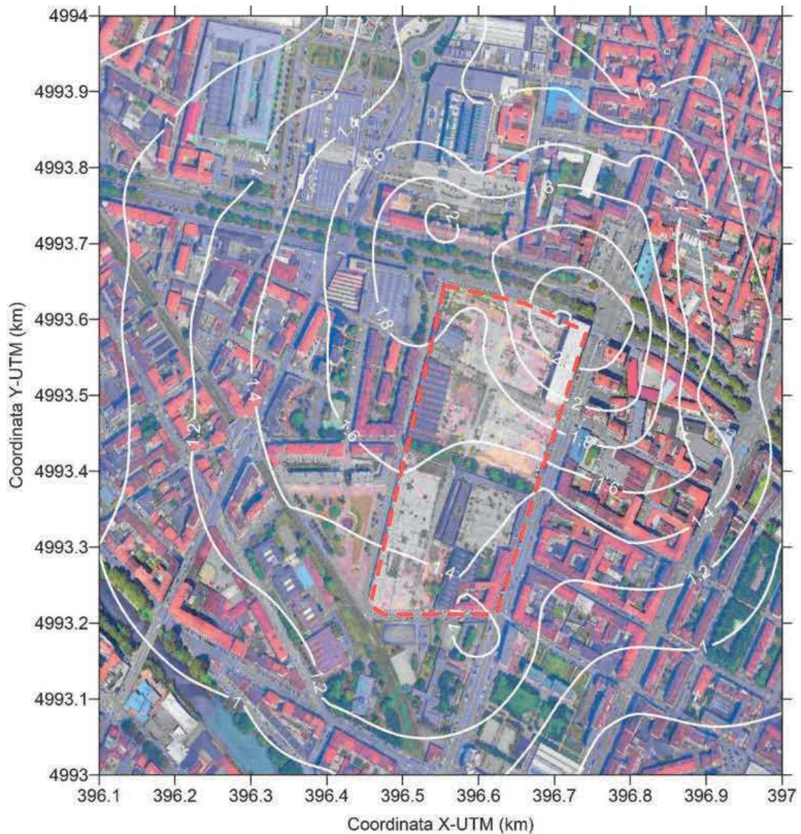
Figura 4-25: Scenario VARIANTE PRIN - Distribuzione spaziale delle concentrazioni massime giornaliere di PM10 (valori in \mu\text{g}/\text{m}^3 )
