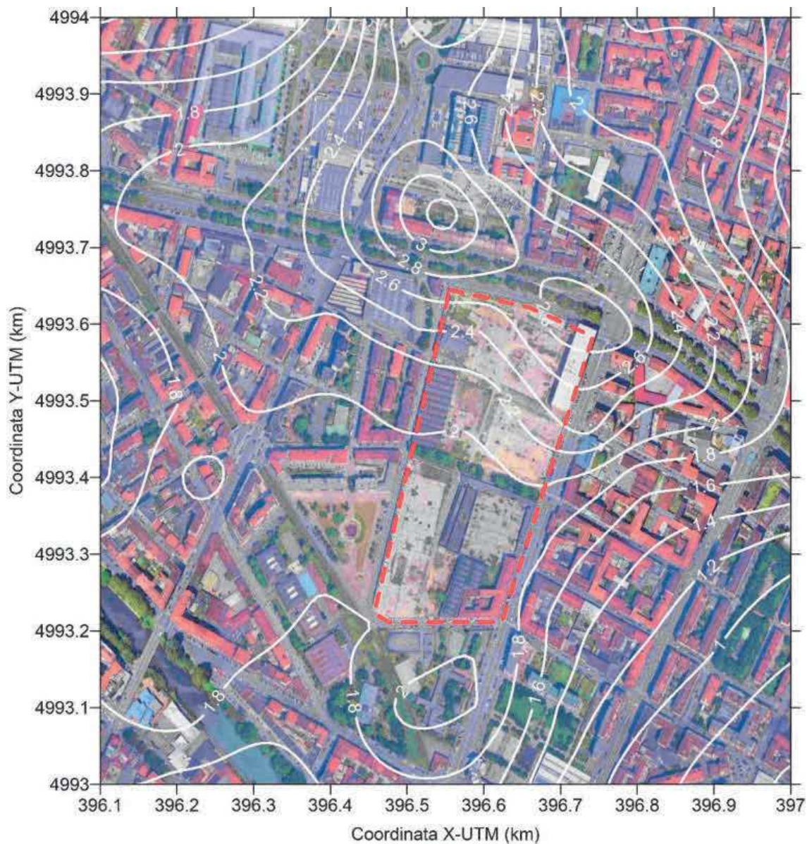
Figura 4-33: Scenario INT - Distribuzione spaziale delle concentrazioni medie annue di PM 2.5 (valori in µg/m 3 )
