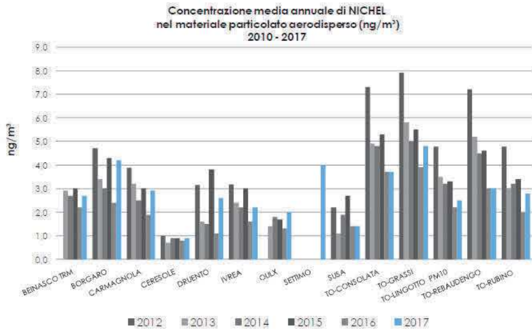
Figura 2-15 Nichel Concentrazione media annua
