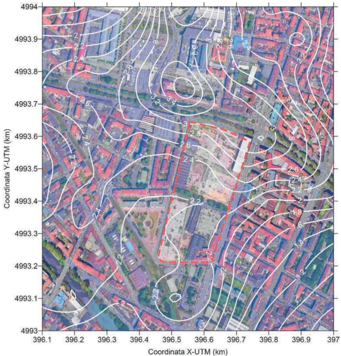
Figura 4-29: Scenario SDF - Distribuzione spaziale delle concentrazioni medie annue di PM10 (valori in \mu\text{g}/\text{m}^3 )
