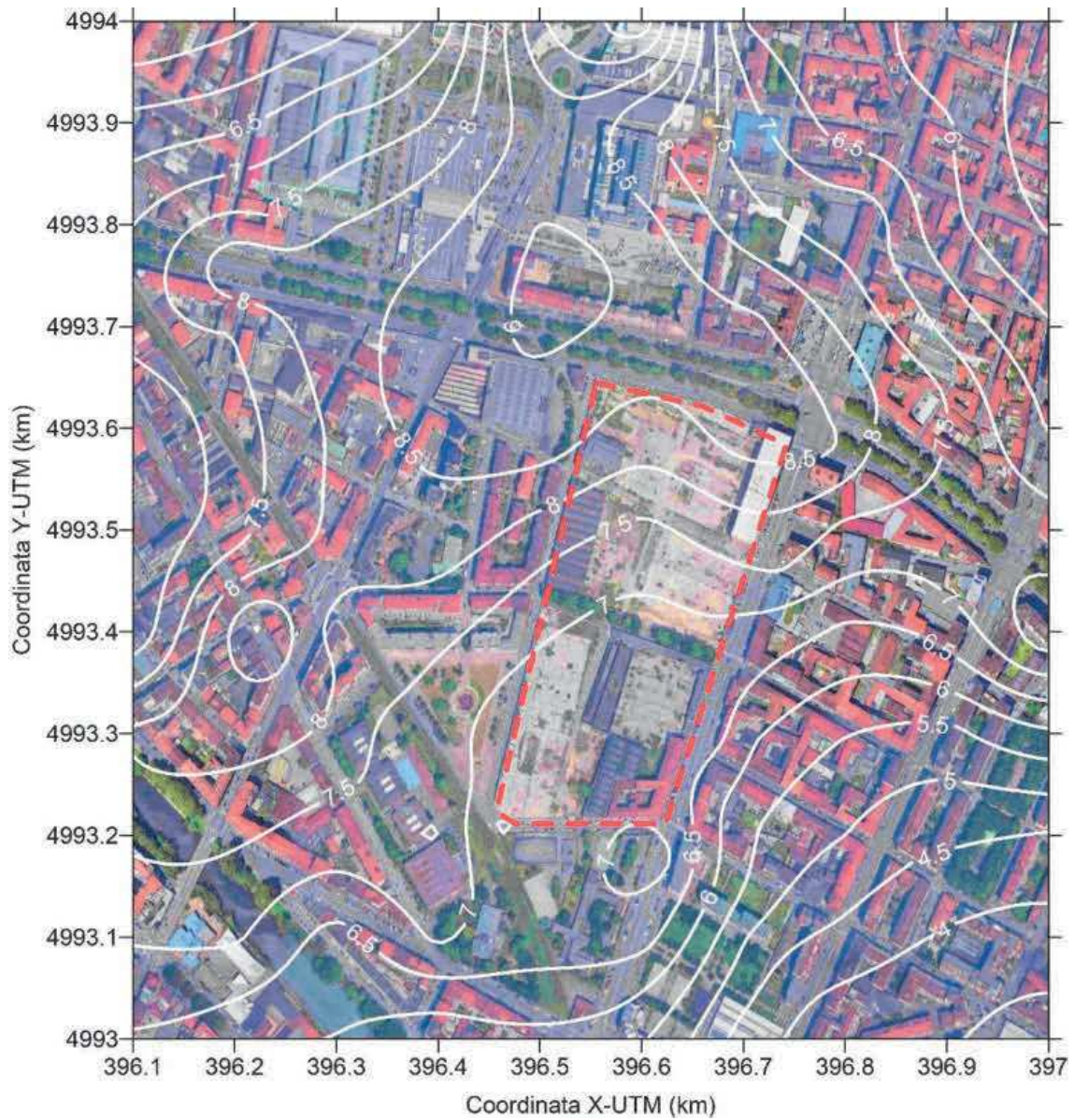
Figura 4-23: Scenario SDF - Distribuzione spaziale delle concentrazioni massime giornaliere di PM10 (valori in \mu\text{g}/\text{m}^3 )
