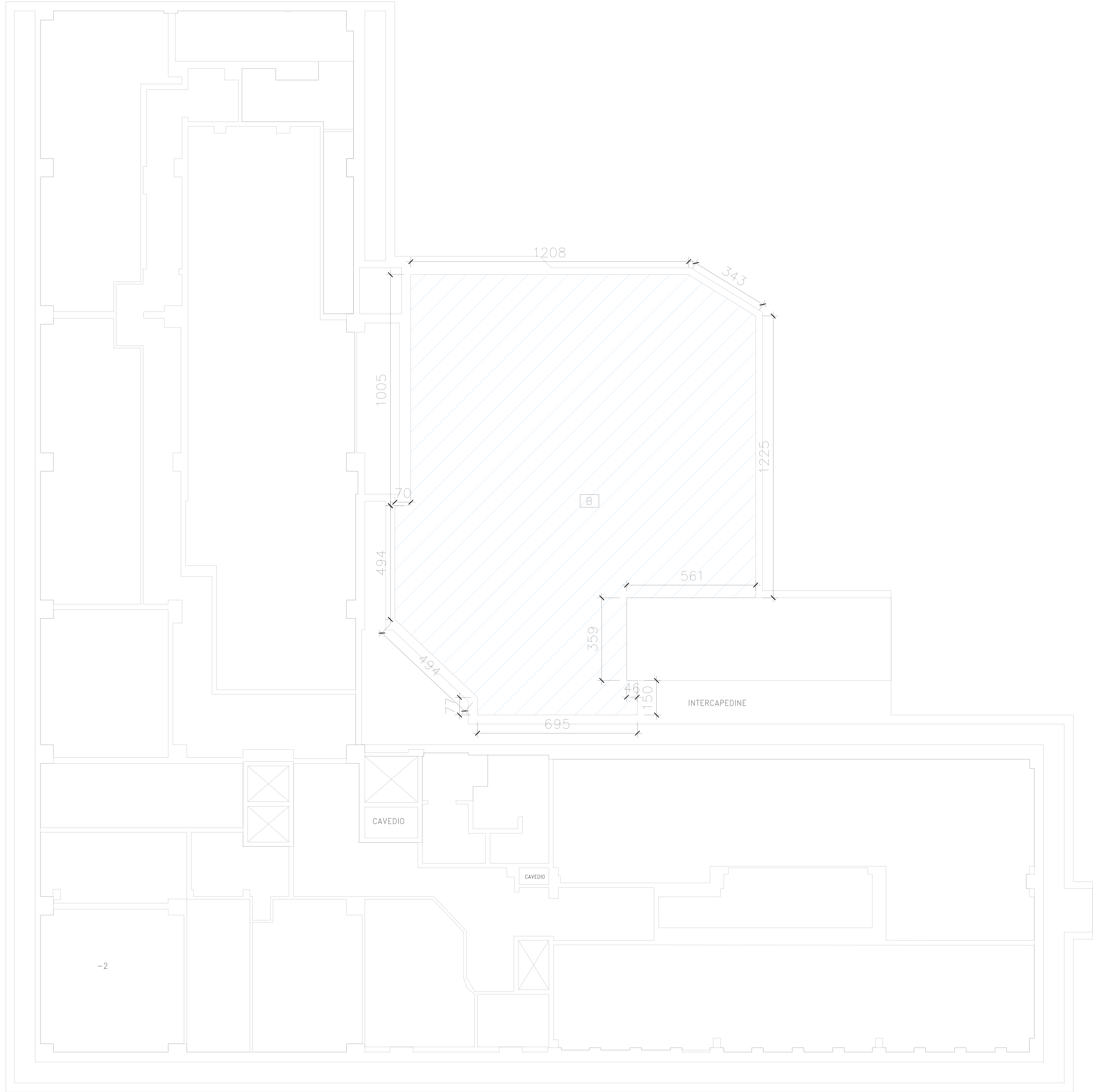
PIANO PRIMO INTERRATO
