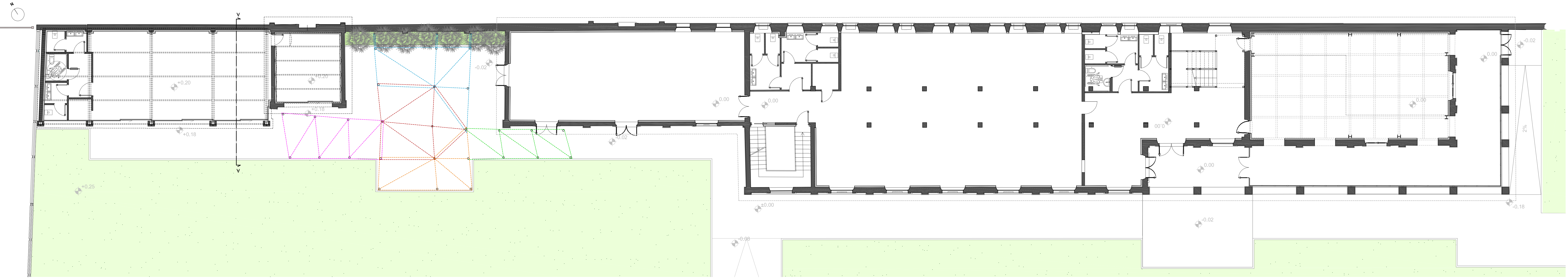
PIANTA PIANO TERRA
