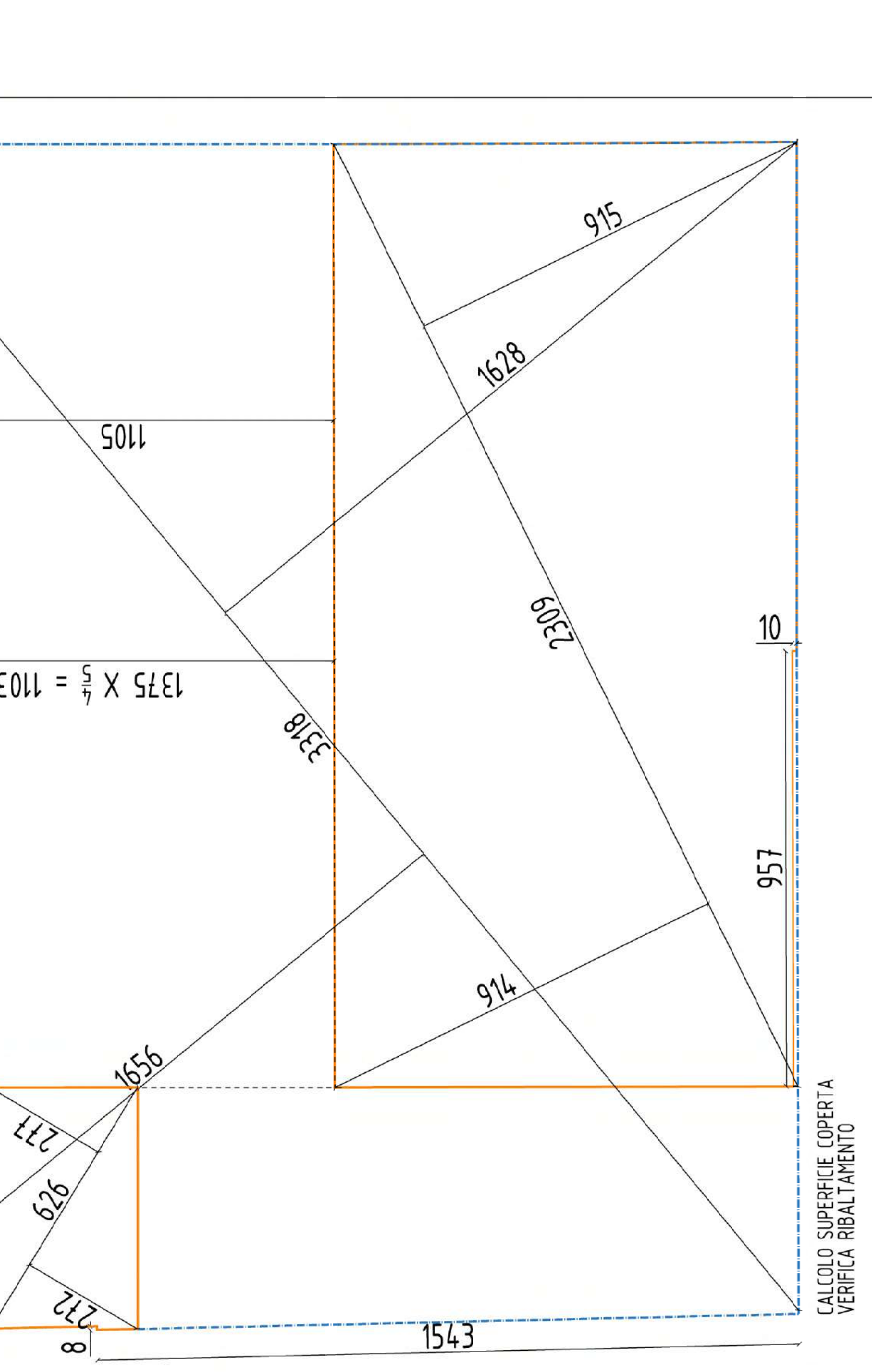
DIMOSTRAZIONE DI CALCOLI DI VERIFICA. SCALA 1:100
