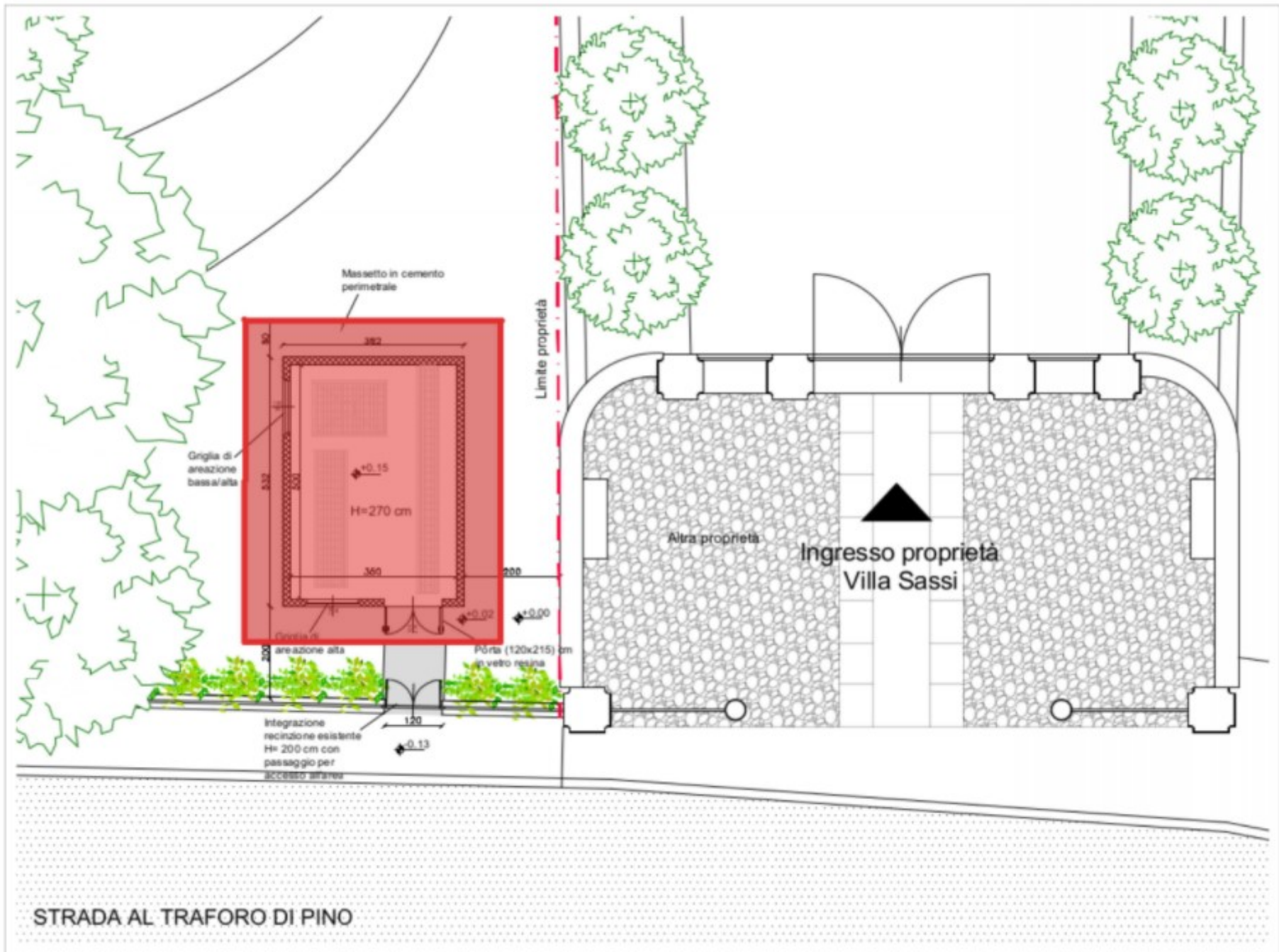
PLANIMETRIA DI PROGETTO
