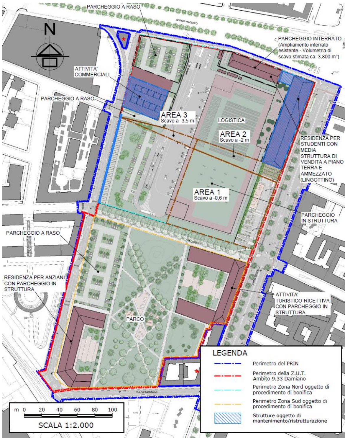
Aree di scavo e relative profondità – Alternativa 2
