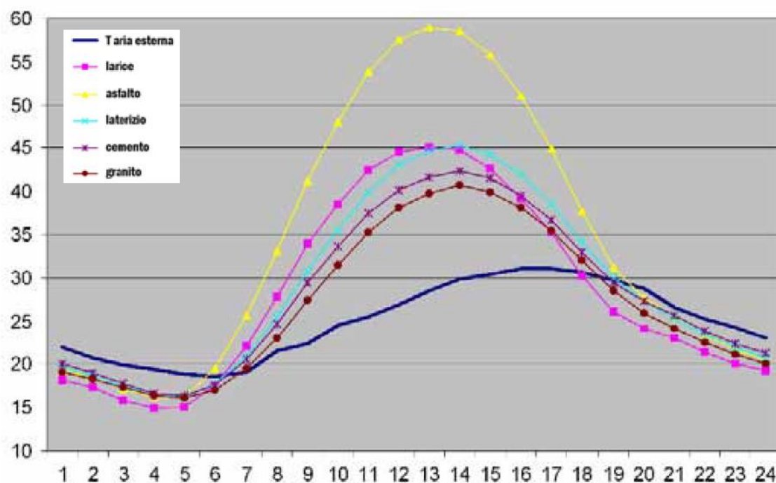
Valori di temperatura superficiale di pavimentazioni realizzate in differenti materiali (asfalto, larice, laterizio, cemento e granito) e temperatura dell'aria esterna 36
