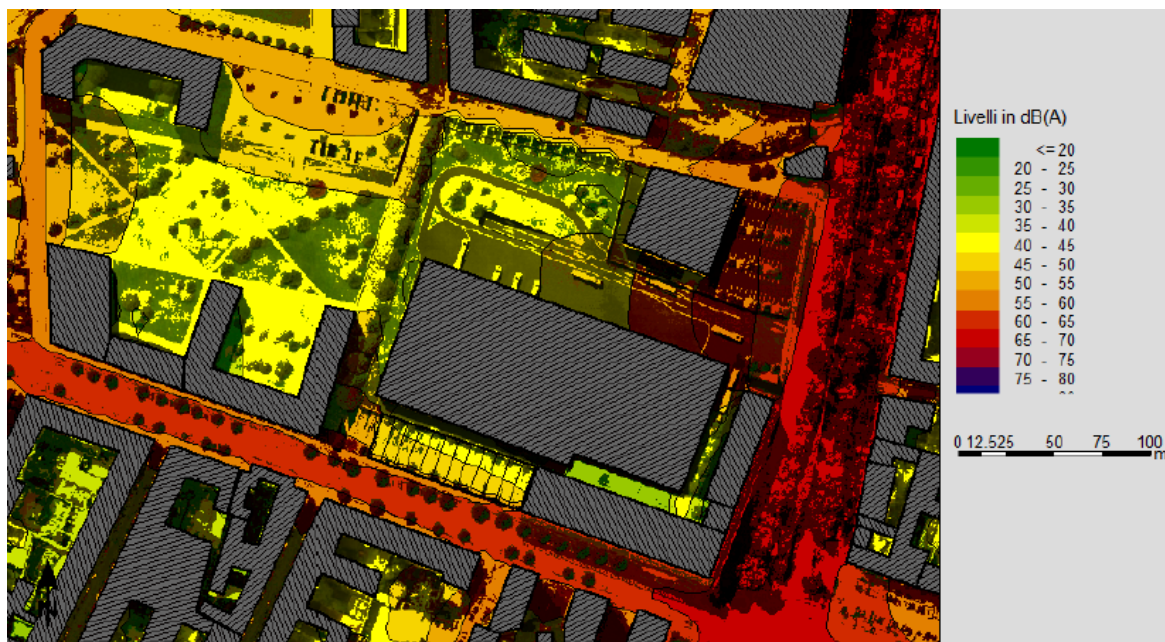
Mapa di rumore stato Post Operam (traffico) – Periodo notturno – quota +4m
