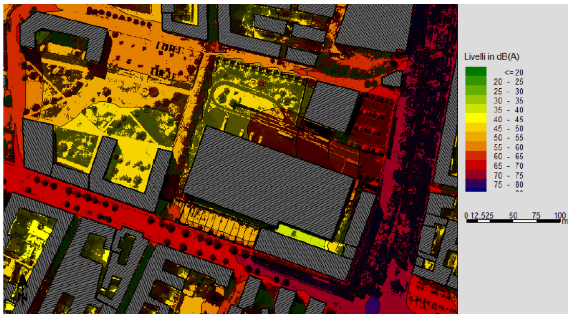
Mapa di rumore stato Post Operam (traffico) – Periodo diurno – quota +4m
