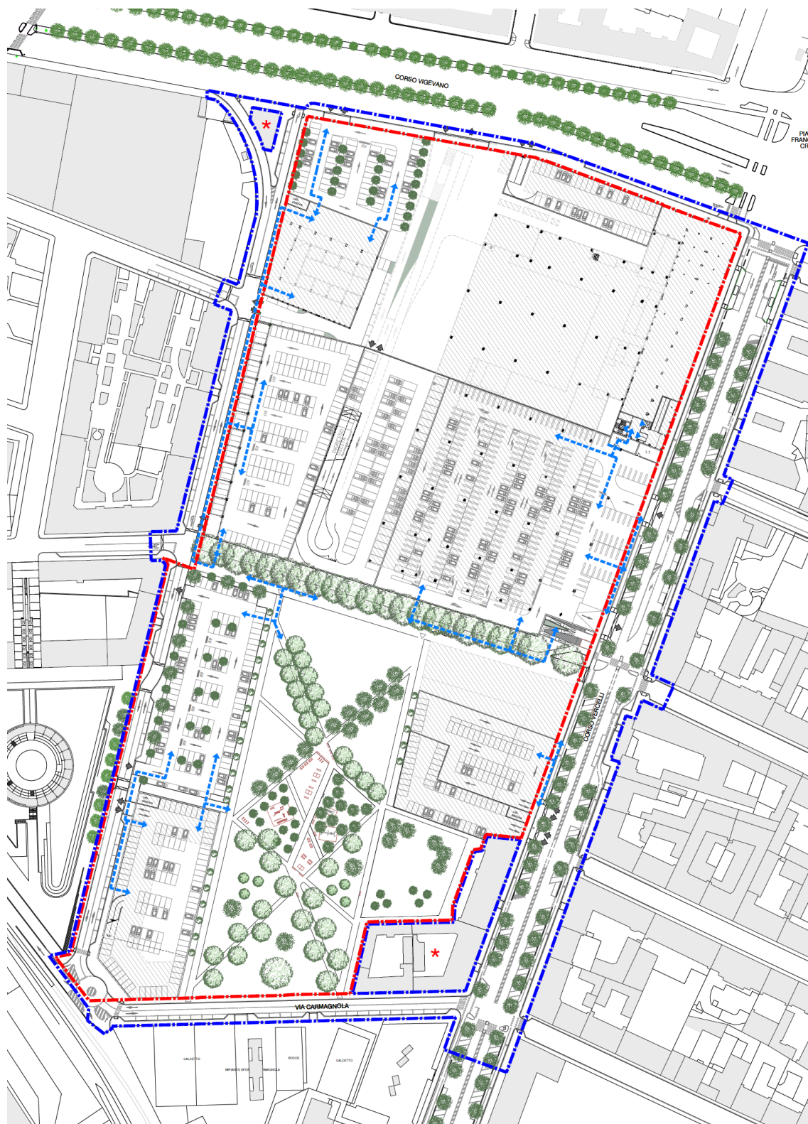
Schema dei collegamenti pedonali dei parcheggi – piano interrato
