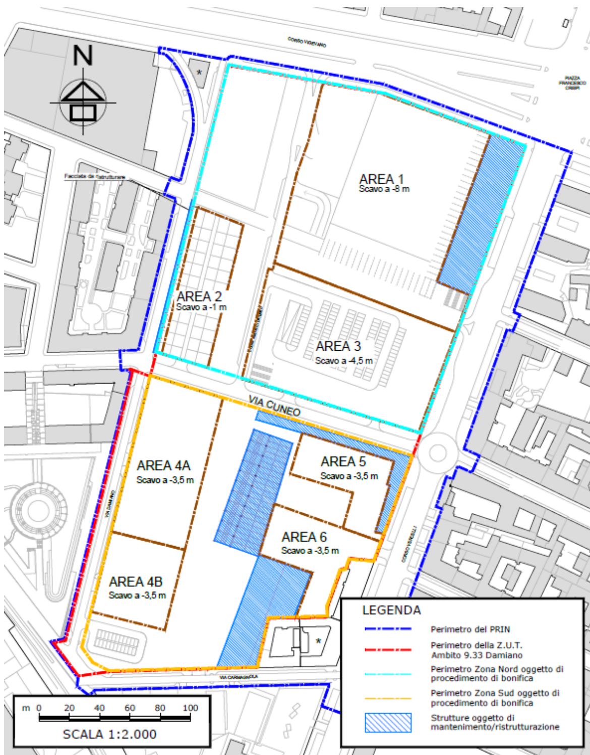
Aree di scavo e relative profondità – Alternativa 3
