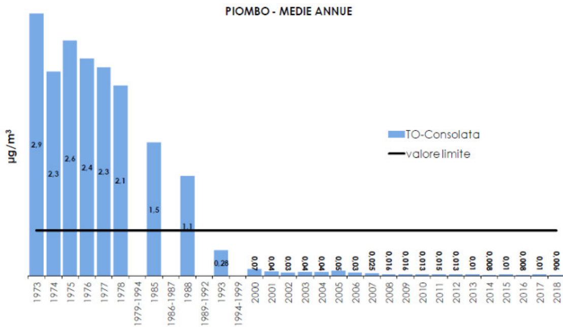
Figura 2-13 Piombo Concentrazione media annua
