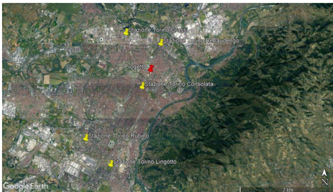
Figura 2-4 Localizzazione delle stazioni di misura
