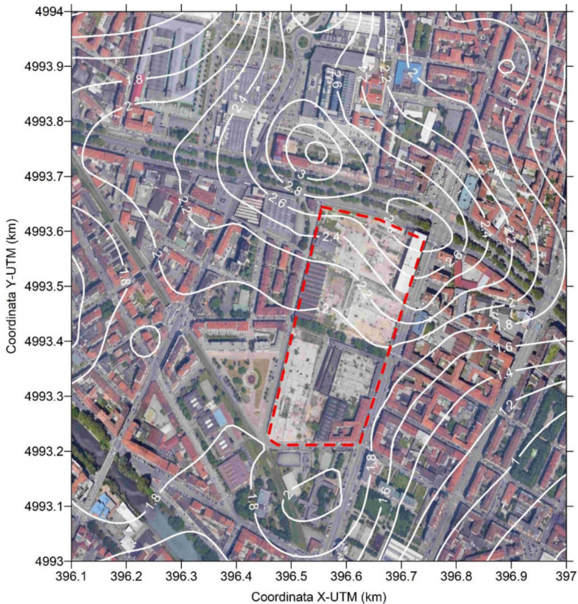
Figura 4-33: Scenario INT - Distribuzione spaziale delle concentrazioni medie annue di PM2.5 (valori in \mu\text{g}/\text{m}^3 )
