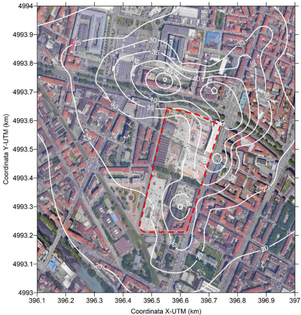
Figura 4-7: Scenario VARIANTE PRIN - Distribuzione spaziale delle concentrazioni massime orarie di NO 2 (valori in \mu\text{g}/\text{m}^3 )
