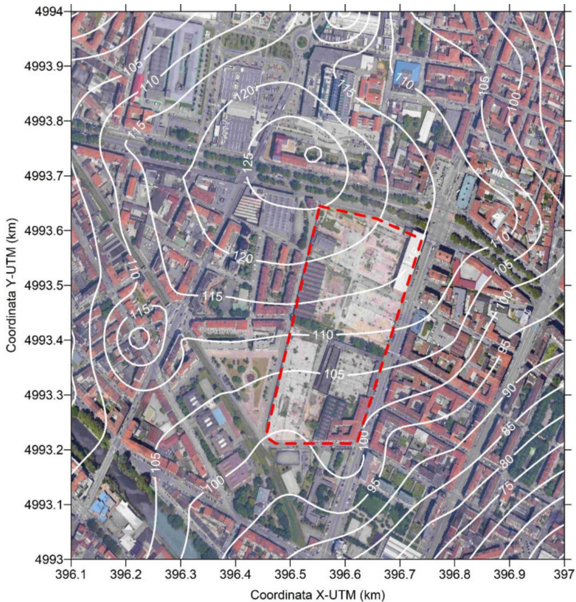
Figura 4-8: Scenario SDF - Distribuzione spaziale del 99.8° percentile delle concentrazioni orarie di NO2 (valori in \mu\text{g}/\text{m}^3 )
