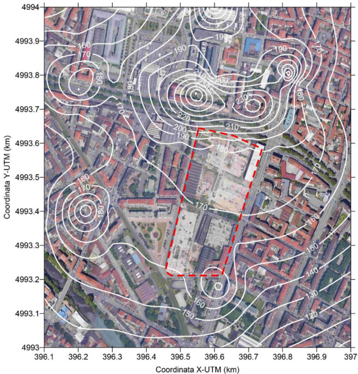
Figura 4-6: Scenario INT - Distribuzione spaziale delle concentrazioni massime orarie di NO 2 (valori in µg/m 3 )
