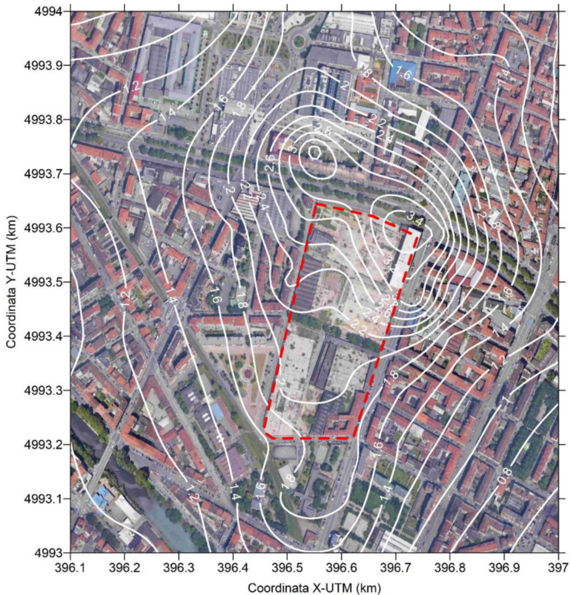
Figura 4-13: Scenario VARIANTE PRIN - Distribuzione spaziale delle concentrazioni medie annue di NO2 (valori in \mu\text{g}/\text{m}^3 )
