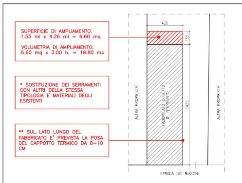
SCHEMA PLANIMETRICO IMMOBILE (PIANO RIALZATO) CON INDICAZIONI DI INTERVENTO – SCALA 1:200
