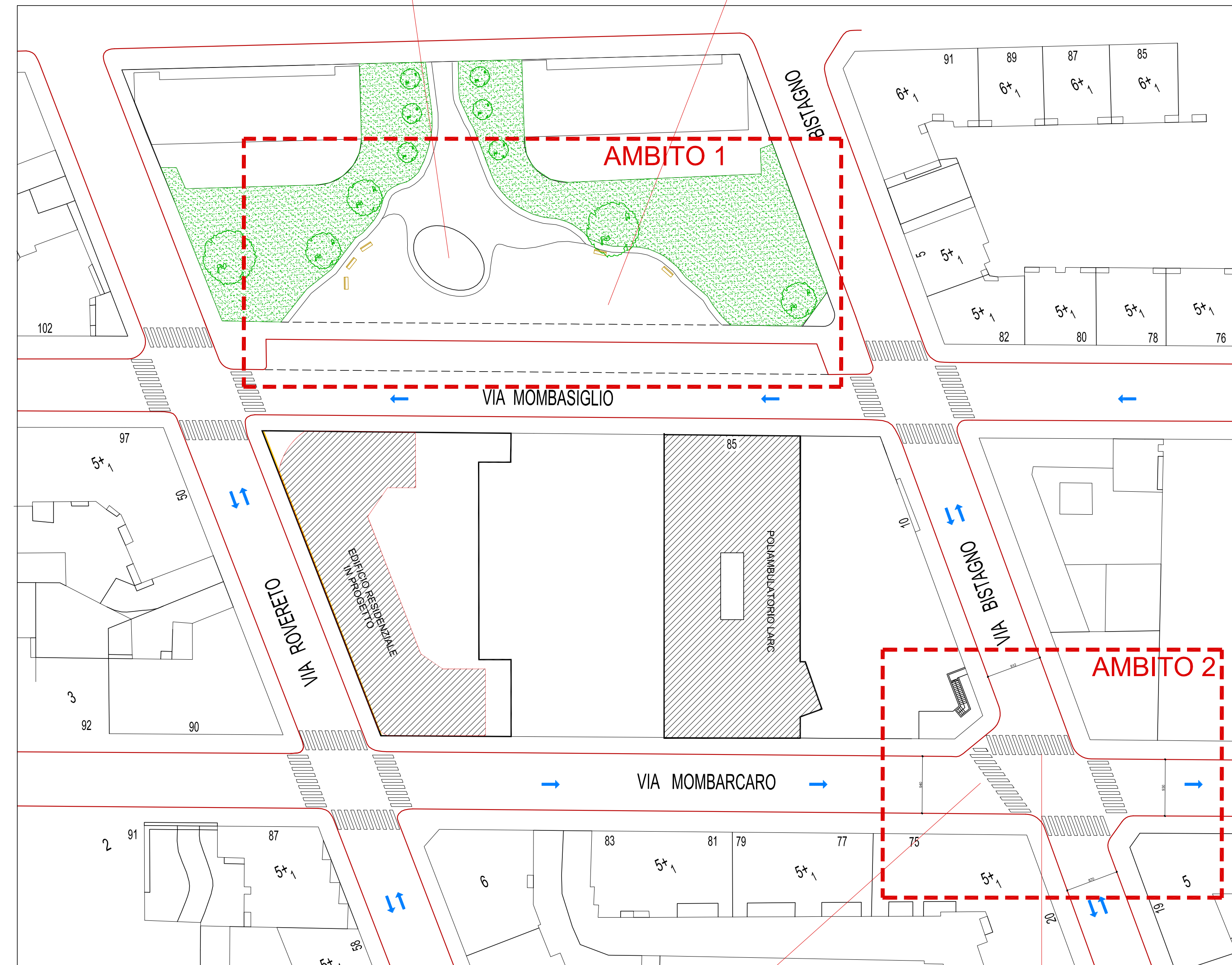
PLANIMETRIA OPERE DI URBANIZZAZIONE STATO DI FATTO
