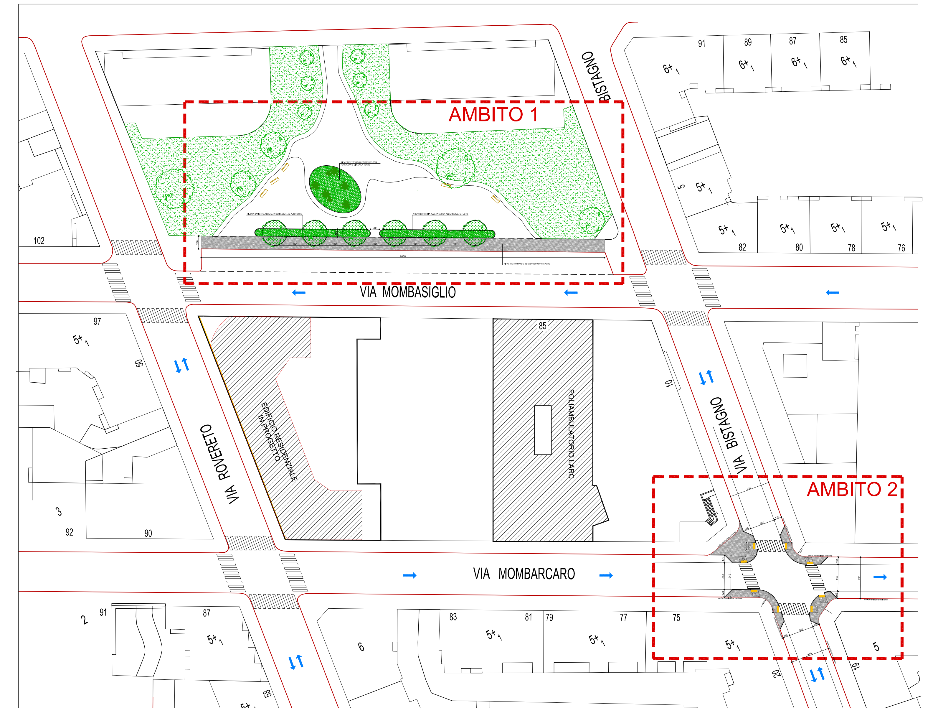
PLANIMETRIA OPERE DI URBANIZZAZIONE PROGETTO
