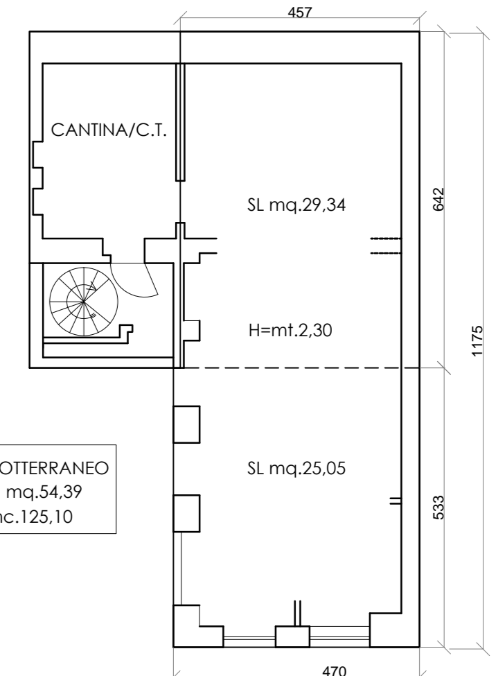
PIANO SOTTERRANEO
