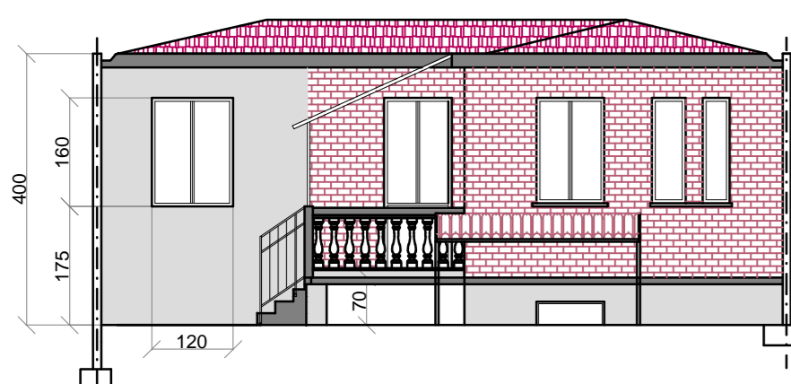
PROSPETTO EST PROPOSTA
