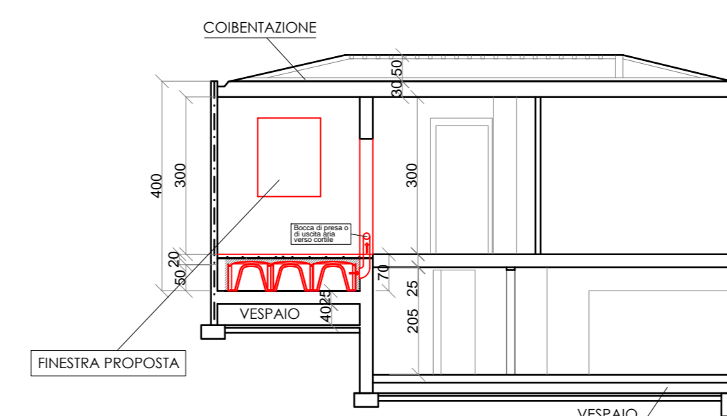
PROPOSTA SEZIONE A-A'
