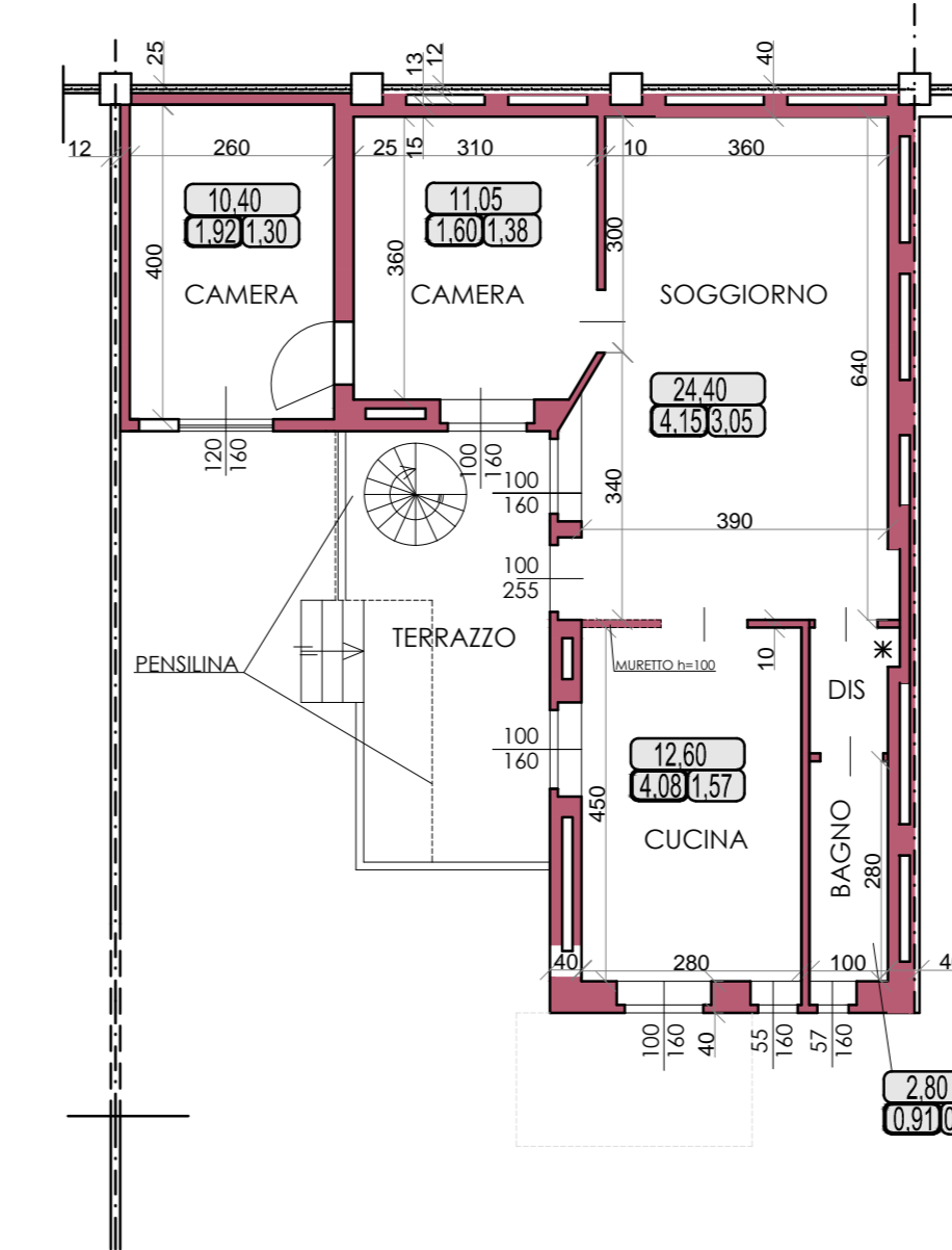
SUPERFICI AEROILLUMINANTI PIANO TERRENO
