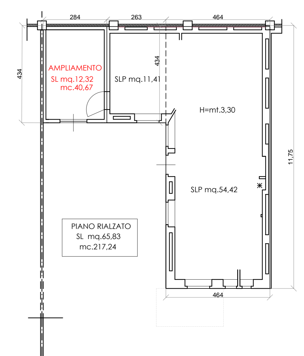
CALCOLO SUPERFICI PIANO TERRENO
