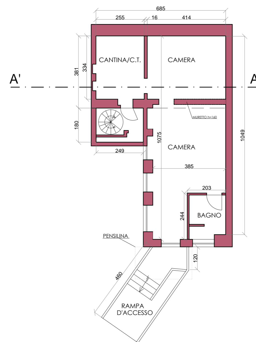
PROPOSTA PIANO SOTTERRANEO INVARIATO
