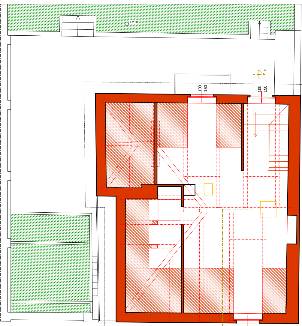
PIANTA PIANO SOTTOTETTO - 1:100
