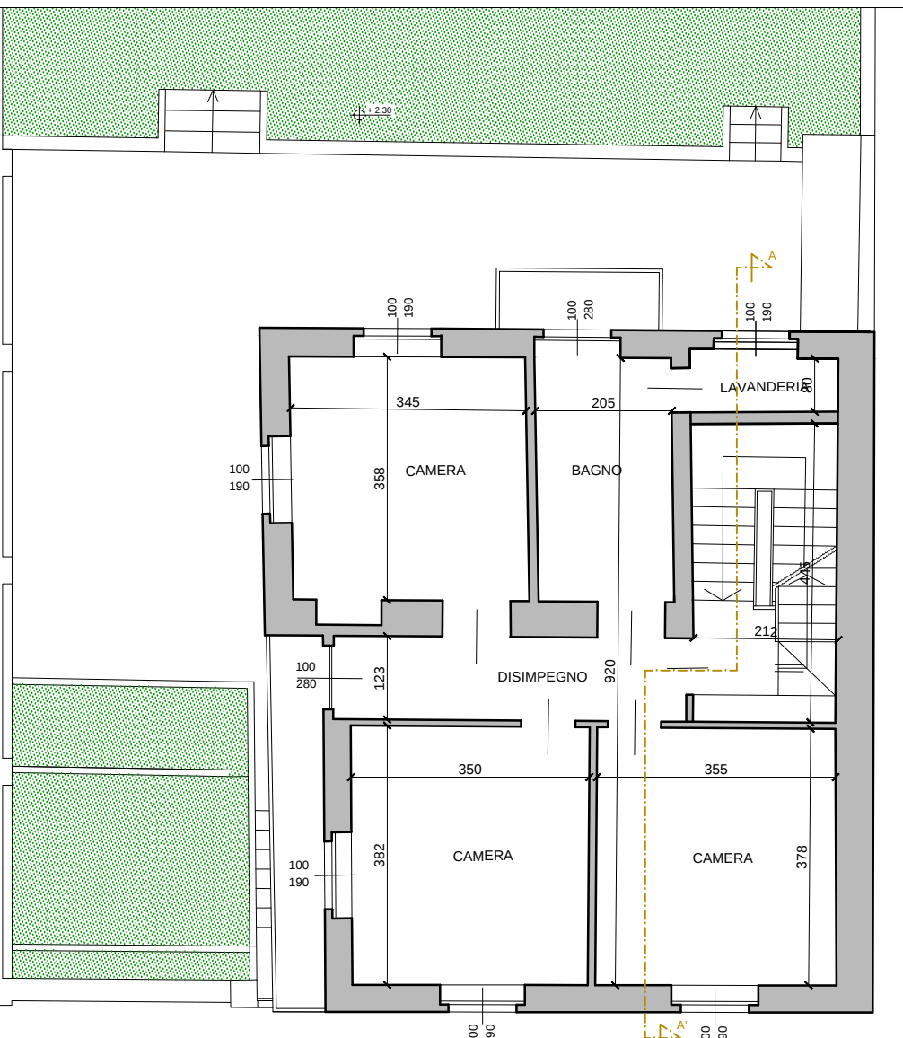
PIANTA PIANO PRIMO - 1:100
