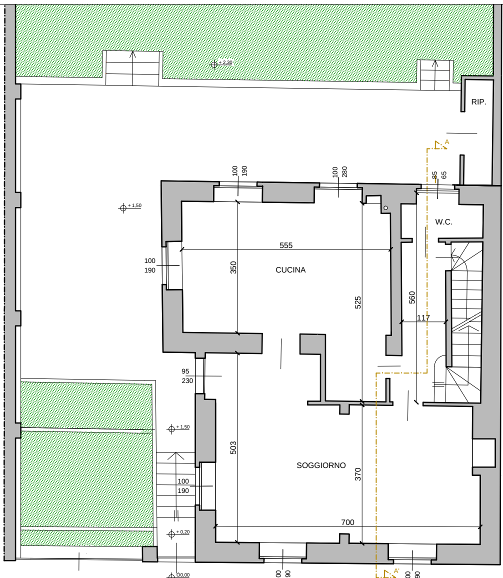
PIANTA PIANO TERRENO - 1:100
