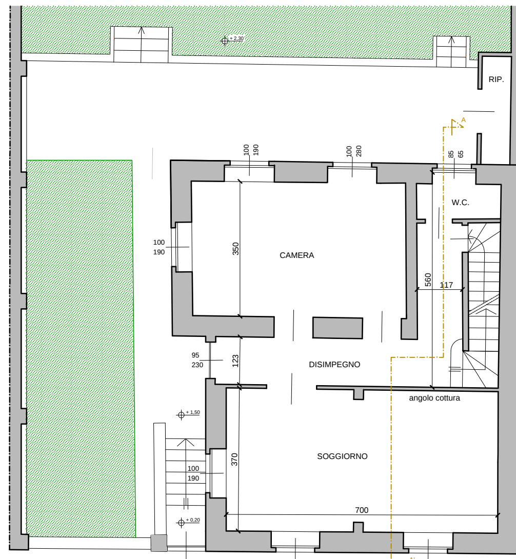
PIANTA PIANO TERRENO - 1:100
