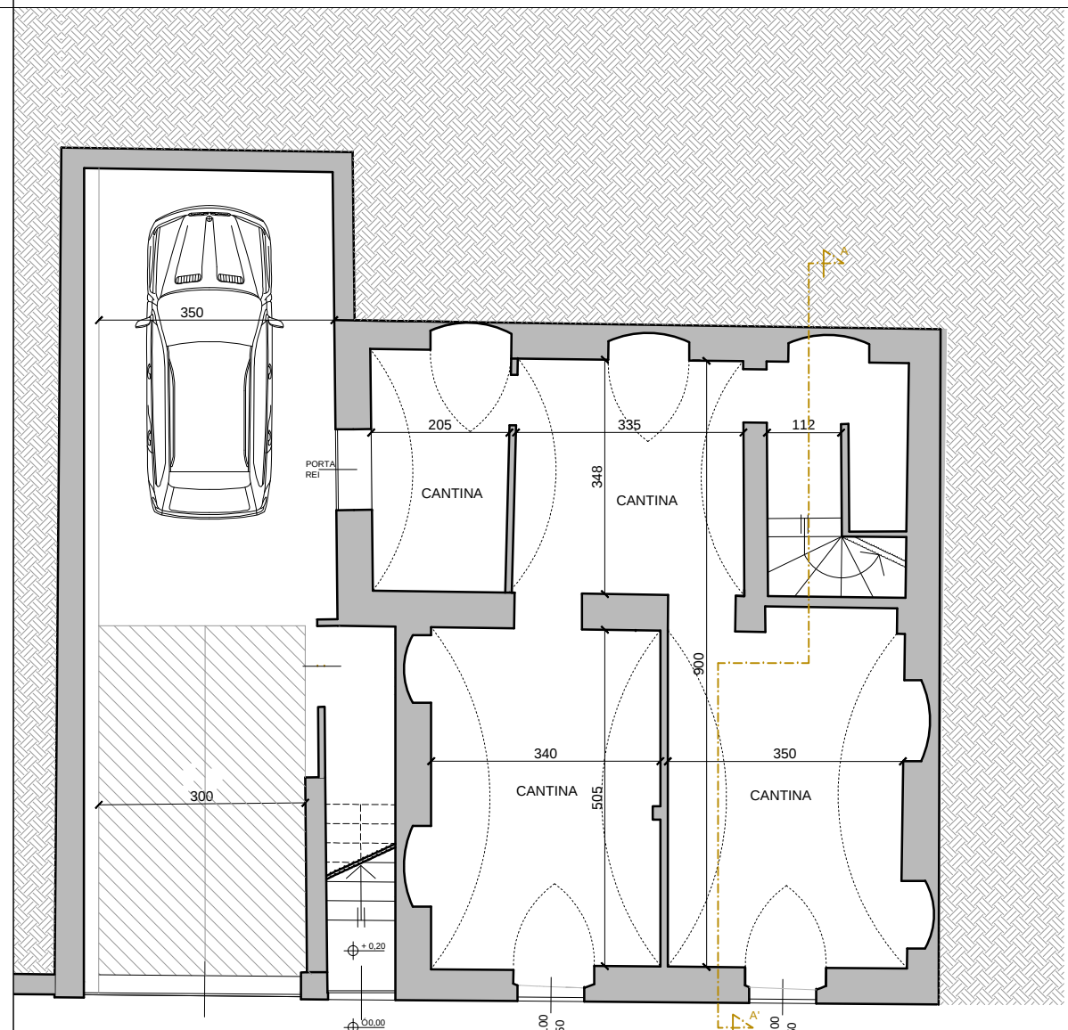
PIANTA PIANO INTERRATO - 1:100
