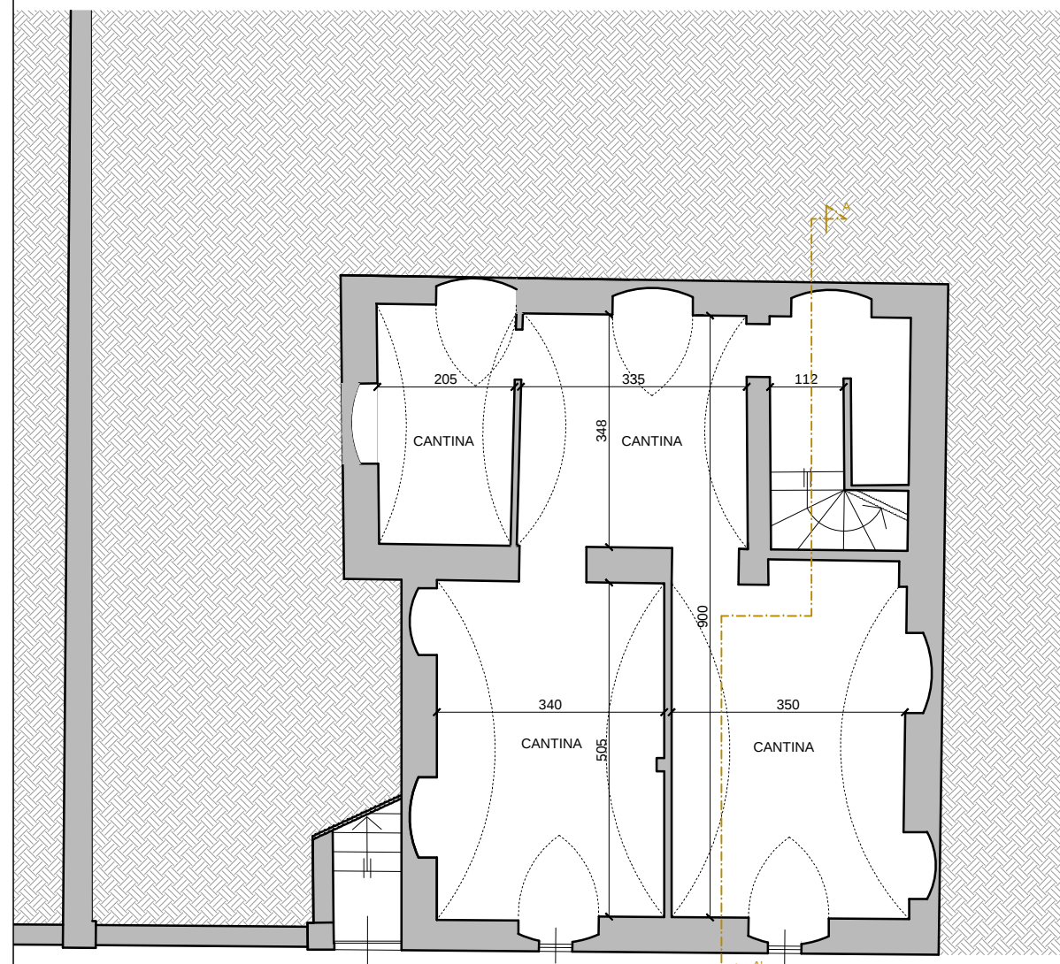
PIANTA PIANO INTERRATO - 1:100
