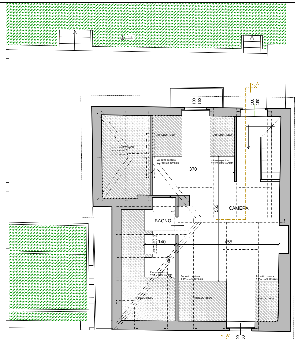
PIANTA PIANO SOTTOTETTO - 1:100
