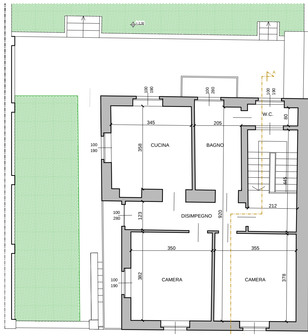
PIANTA PIANO PRIMO - 1:100
