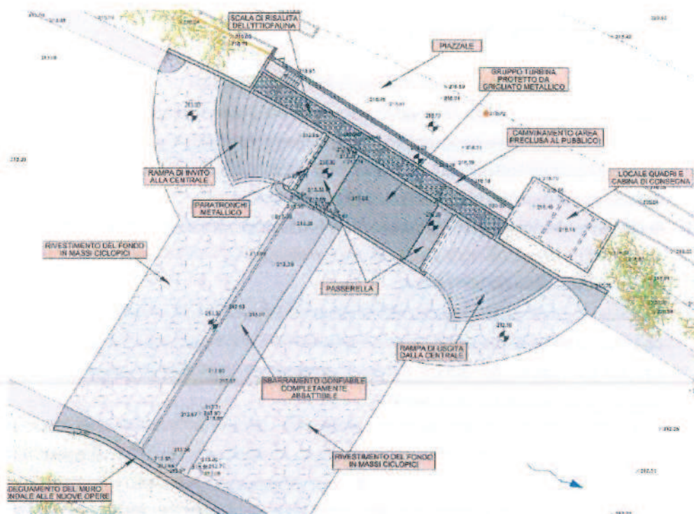
Figura 2 – Planimetria della derivazione
