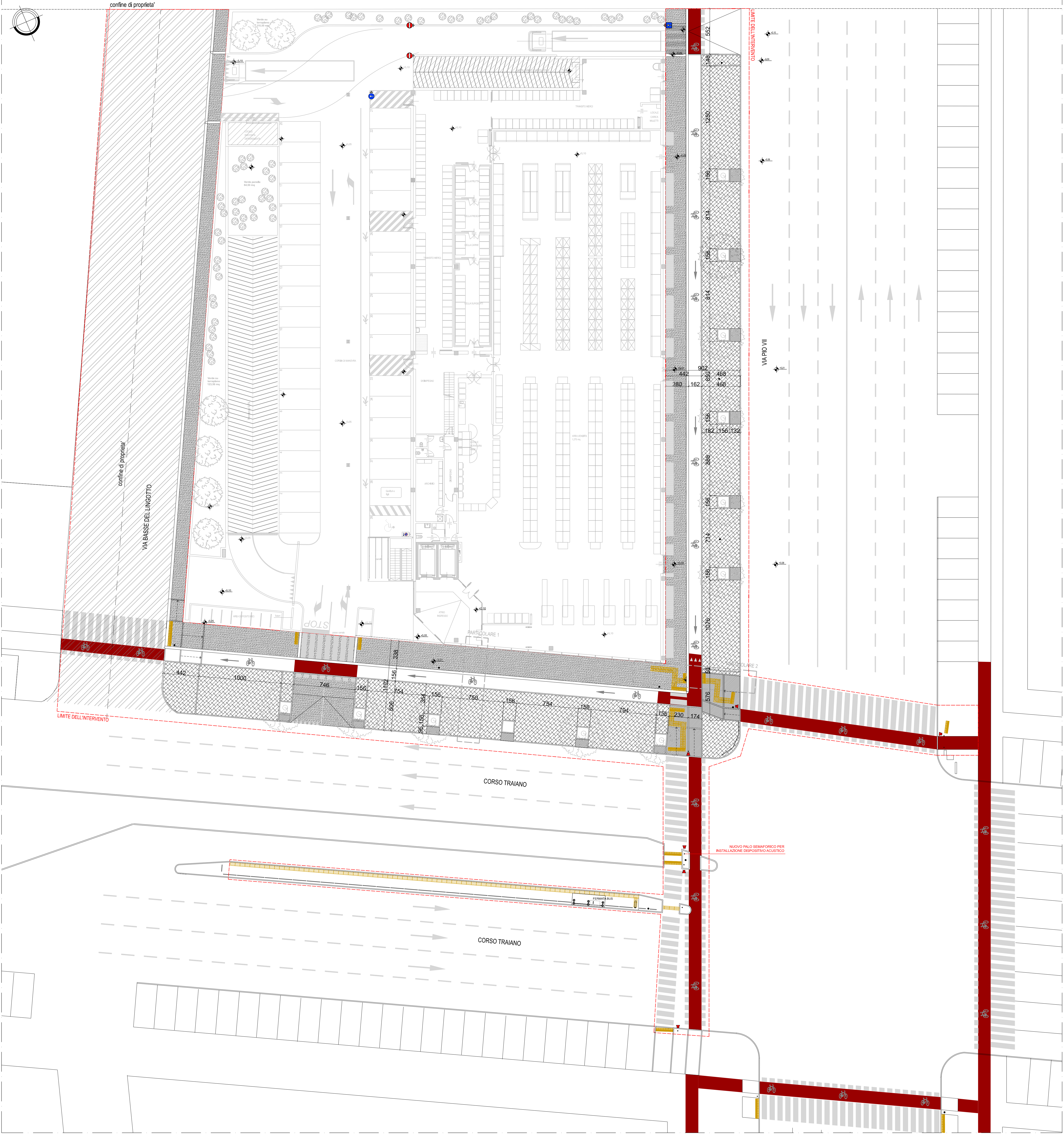
PLANIMETRIA GENERALE - SCALA 1:200
