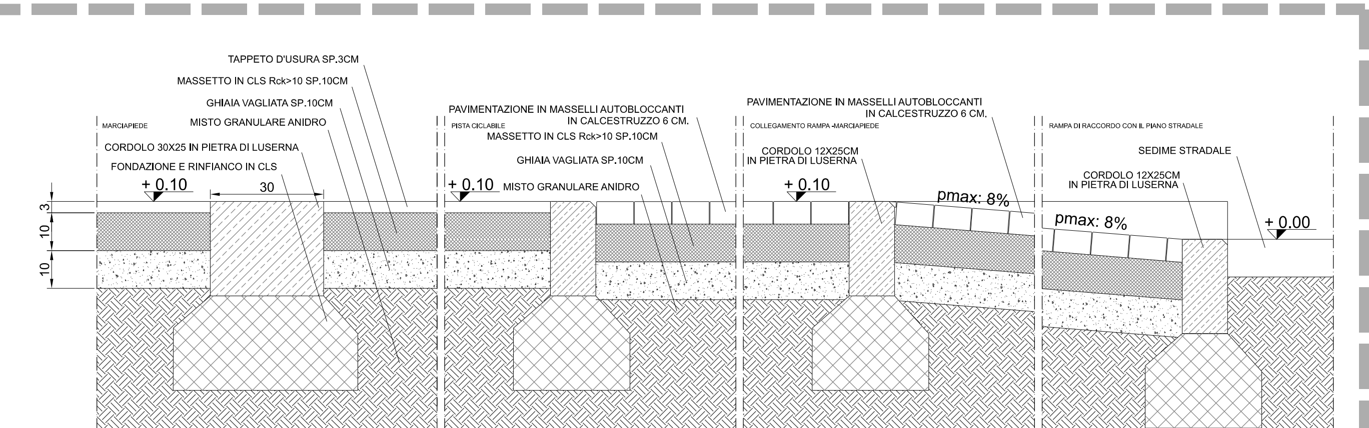
PARTICOLARE 2 - SCALA 1:10
