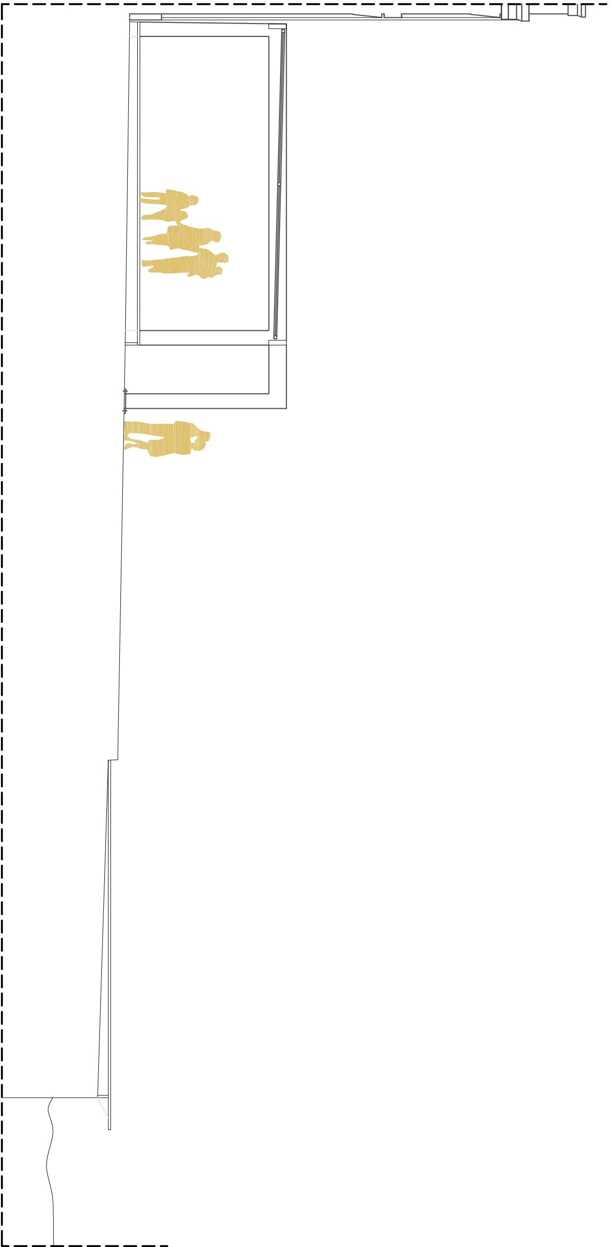
SEZIONE TRASVERSALE - STRUTTURE ESTERNE IN FASE DI CHIUSURA DEI LOCALI
