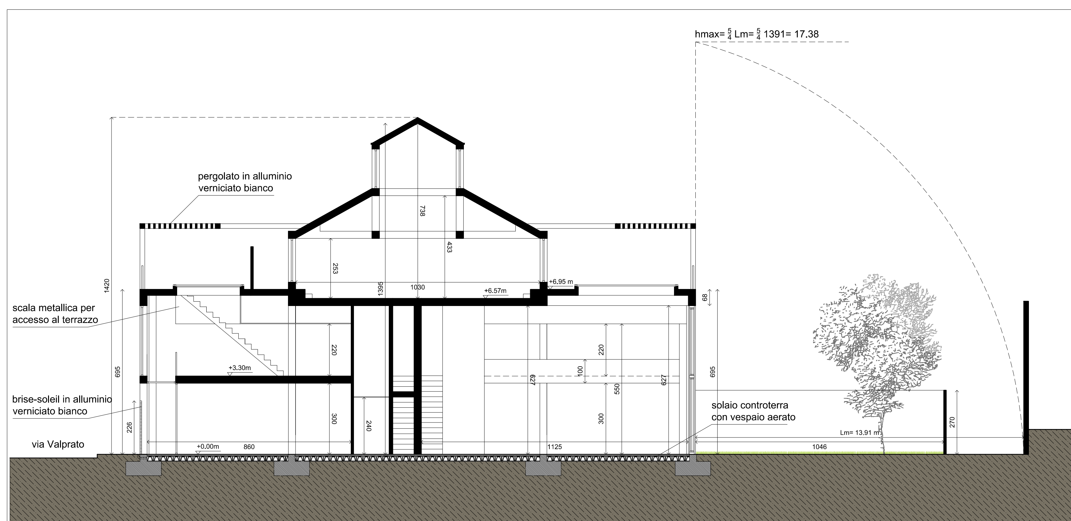
SEZIONE BB
