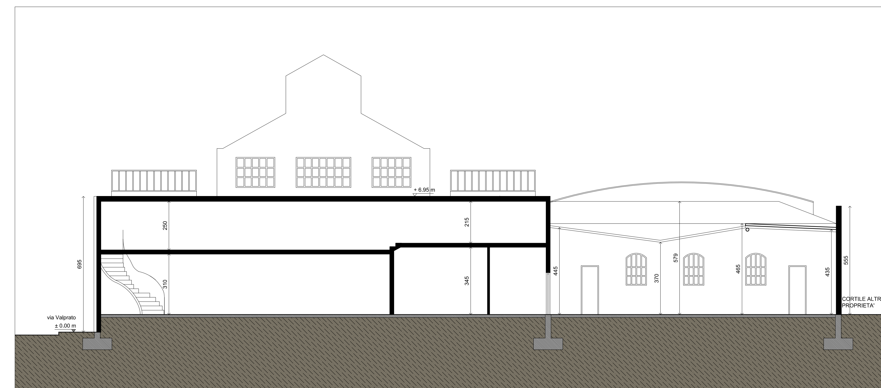
SEZIONE DD
