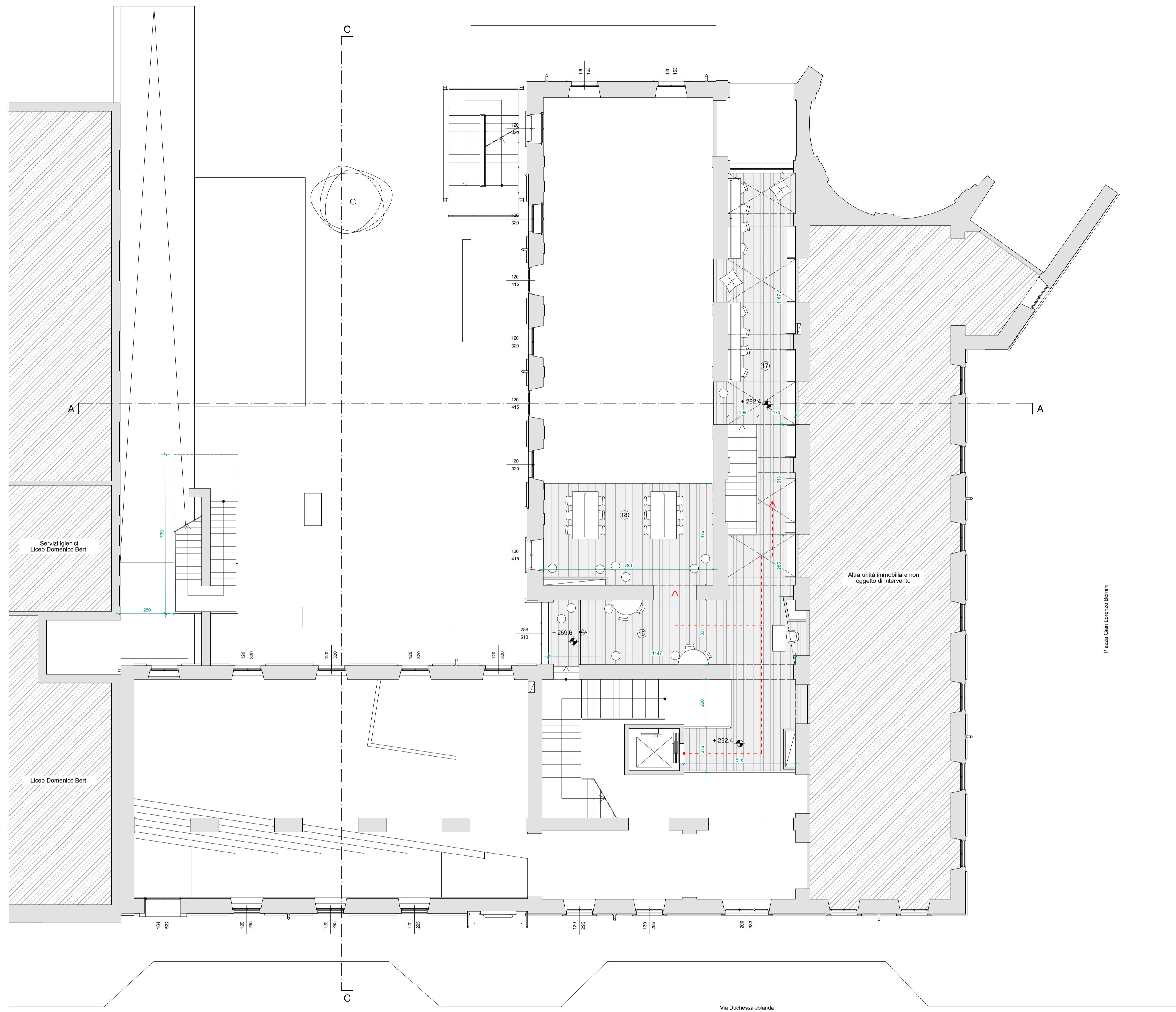
PIANTA PIANO PRIMO AMMEZZATO _ SITUAZIONE DI PROGETTO
