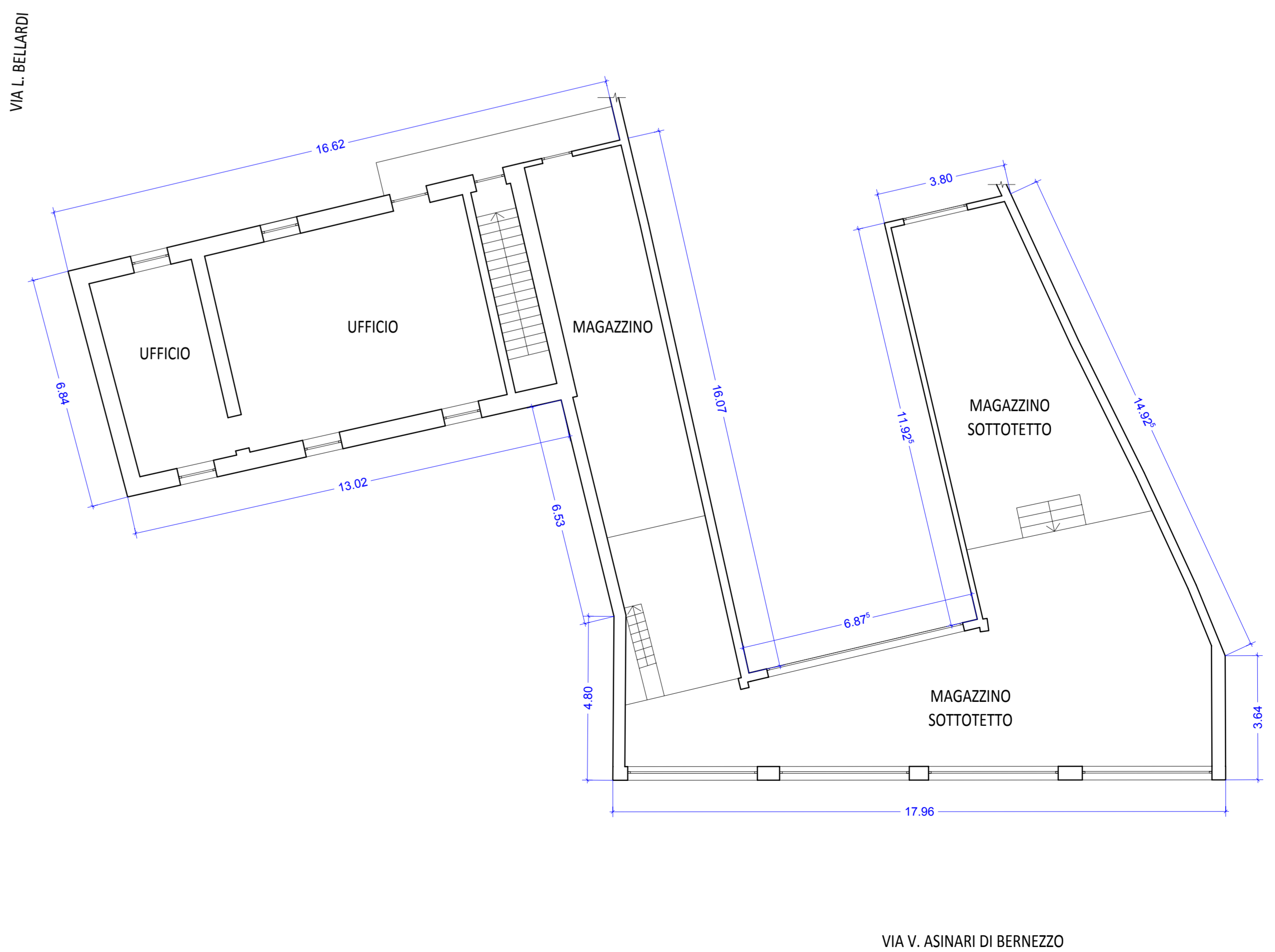
PIANTA PIANO PRIMO 1:100
