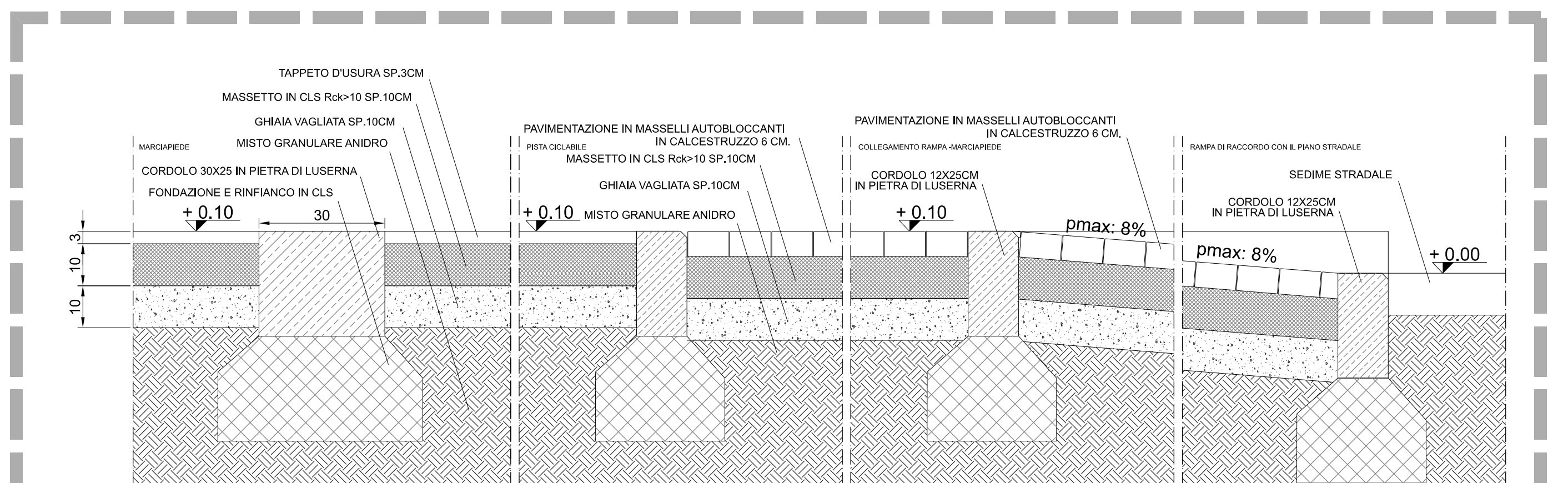
PARTICOLARE 2 - SCALA 1:10
