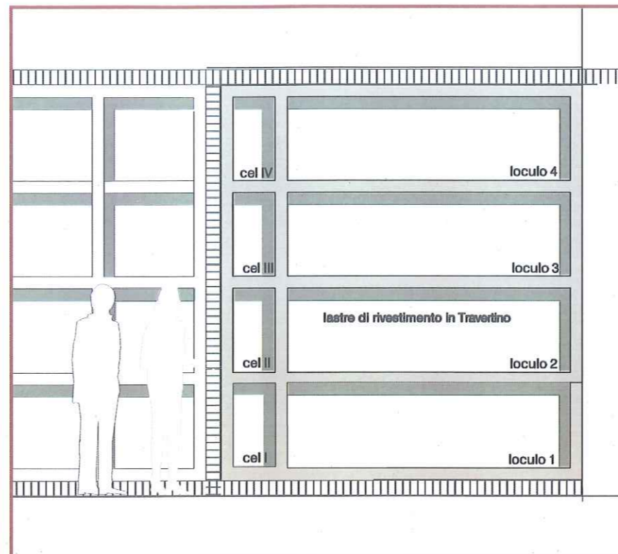
prospetto
