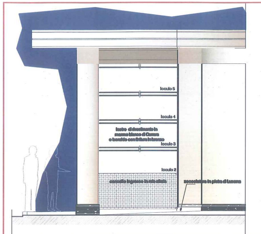
prospetto vista A
