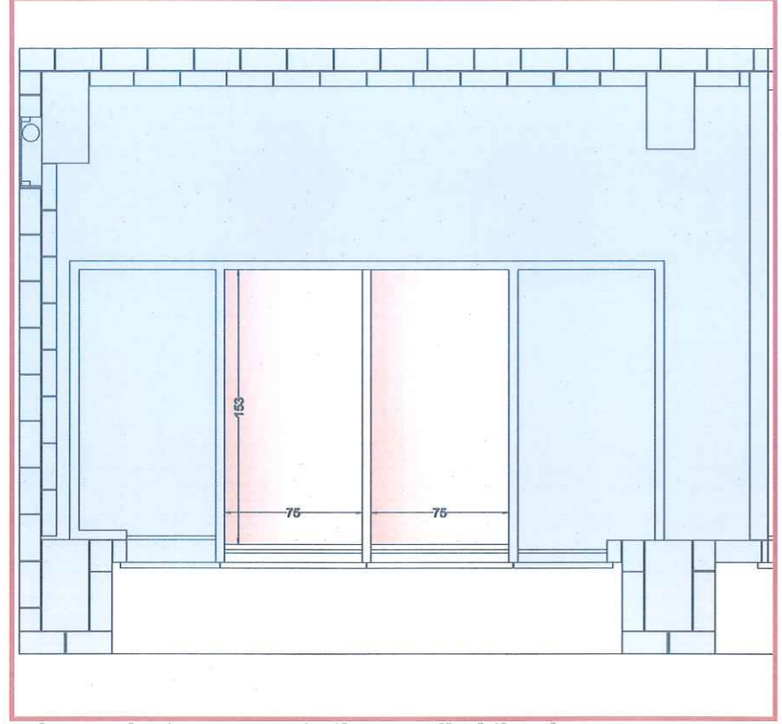
schema pianta scomparto tipo - cellari tipo 1 stato di fatto
