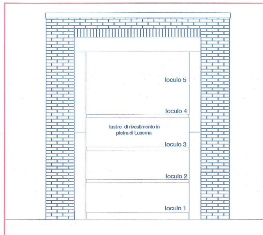
prospetto
