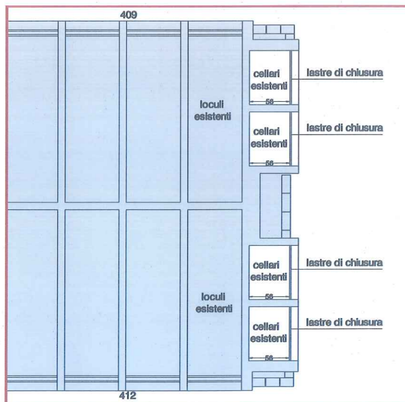
schema pianta scomparto tipo B - piano terra stato di fatto
