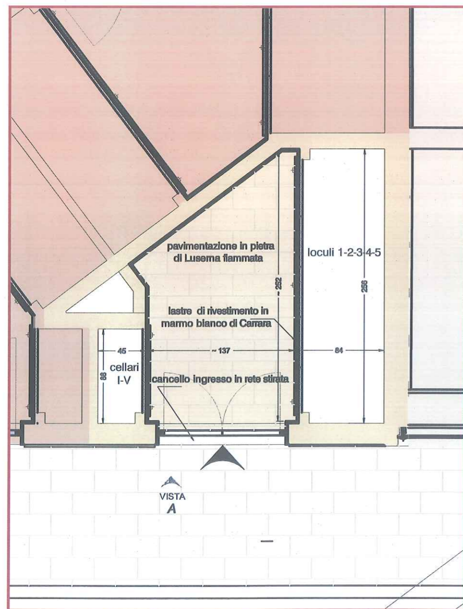
pianta TF4 -TF 6
