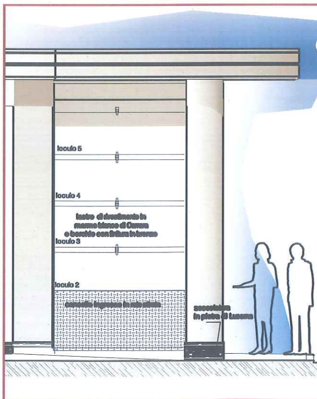
prospetto vista A
