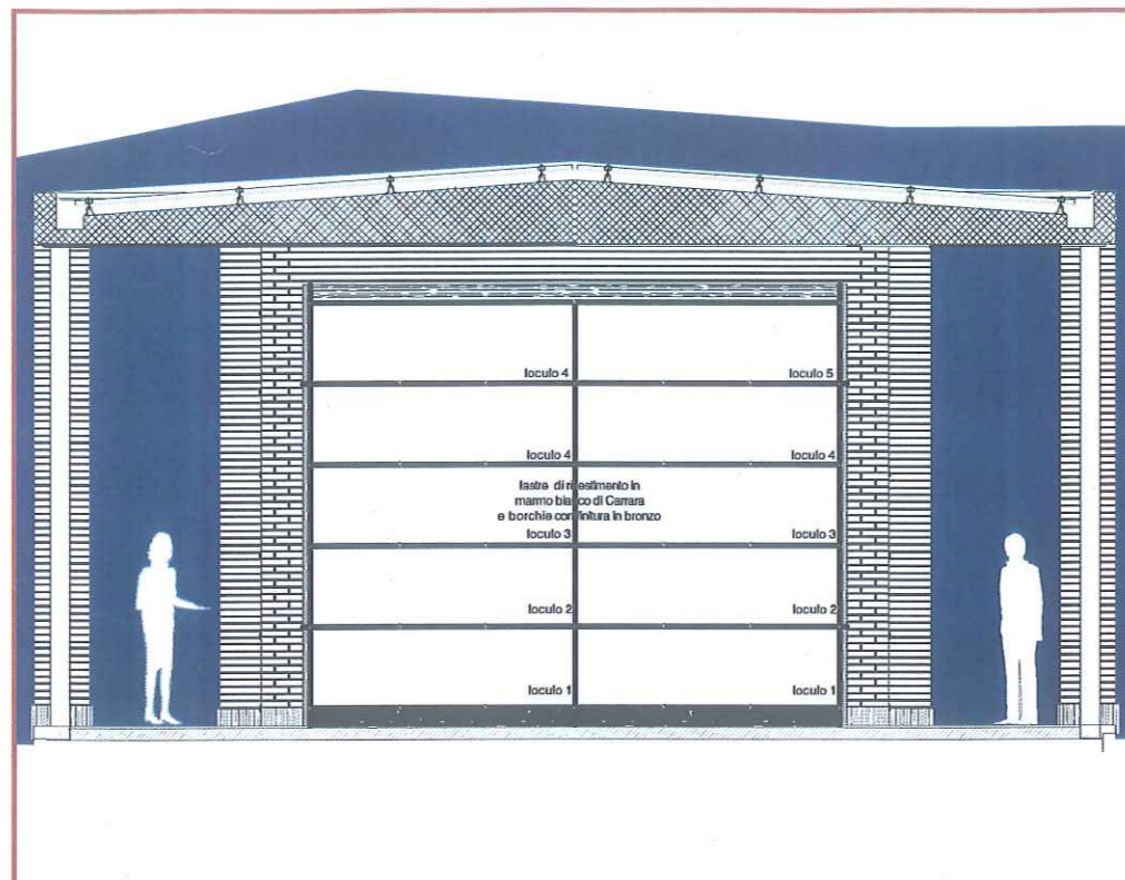
prospetto
