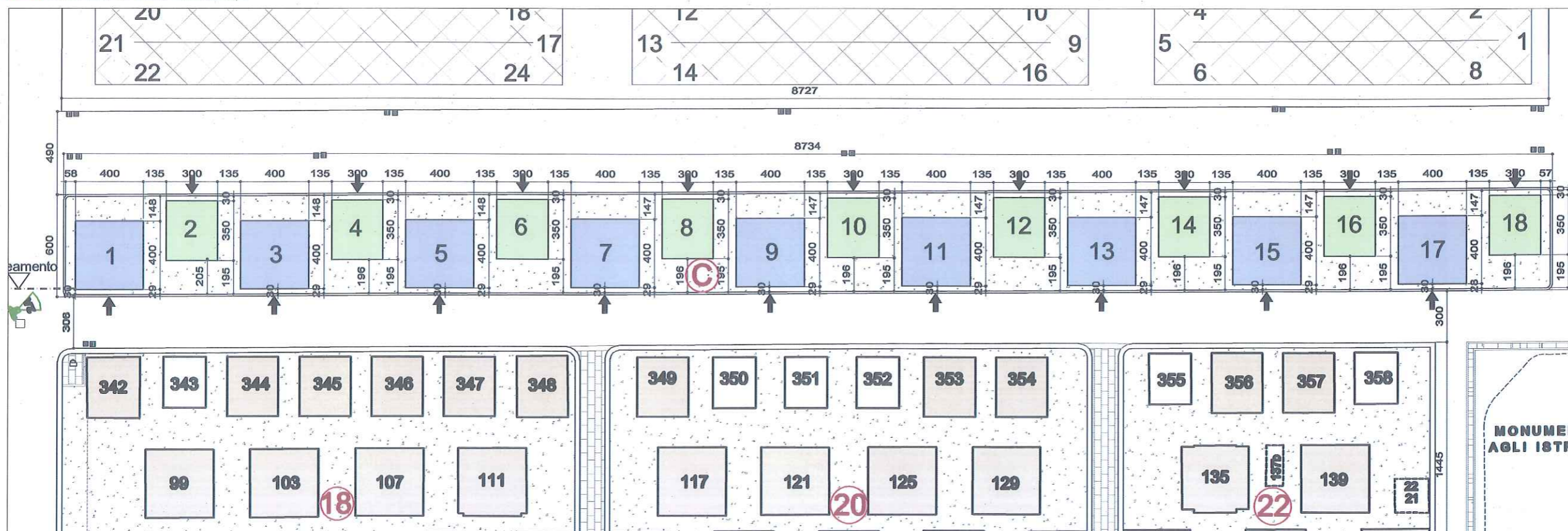
planimetria area per lottizzazione scala 1:250
