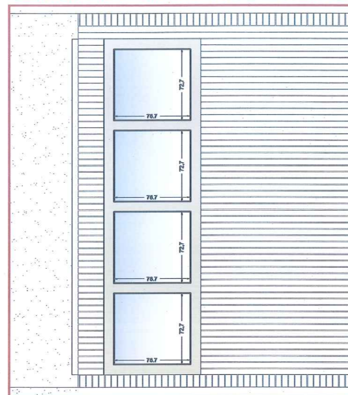
schema prospetto scomparto tipo A - piano primo stato di fatto
