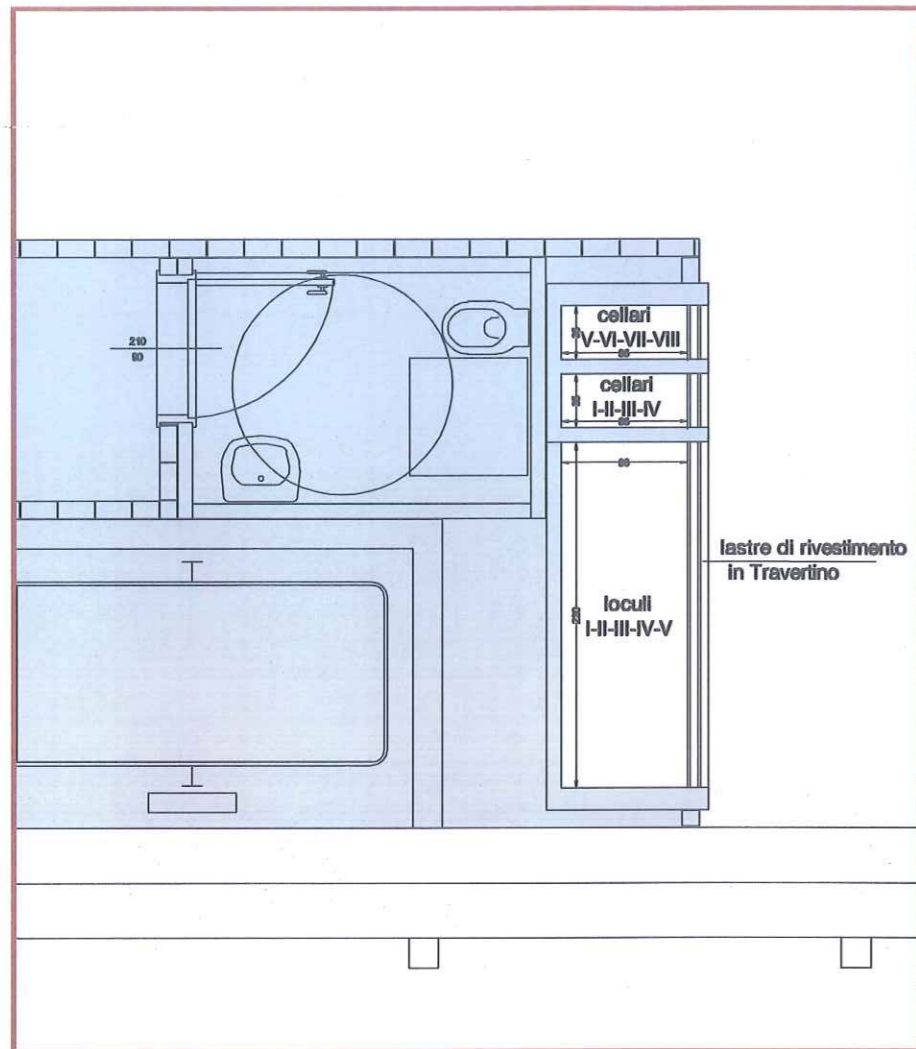
pianta TF10
