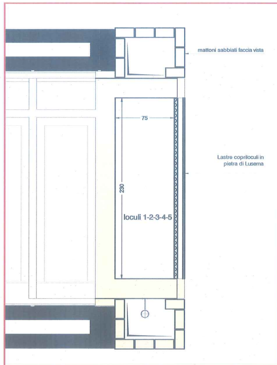
pianta TF tipo
