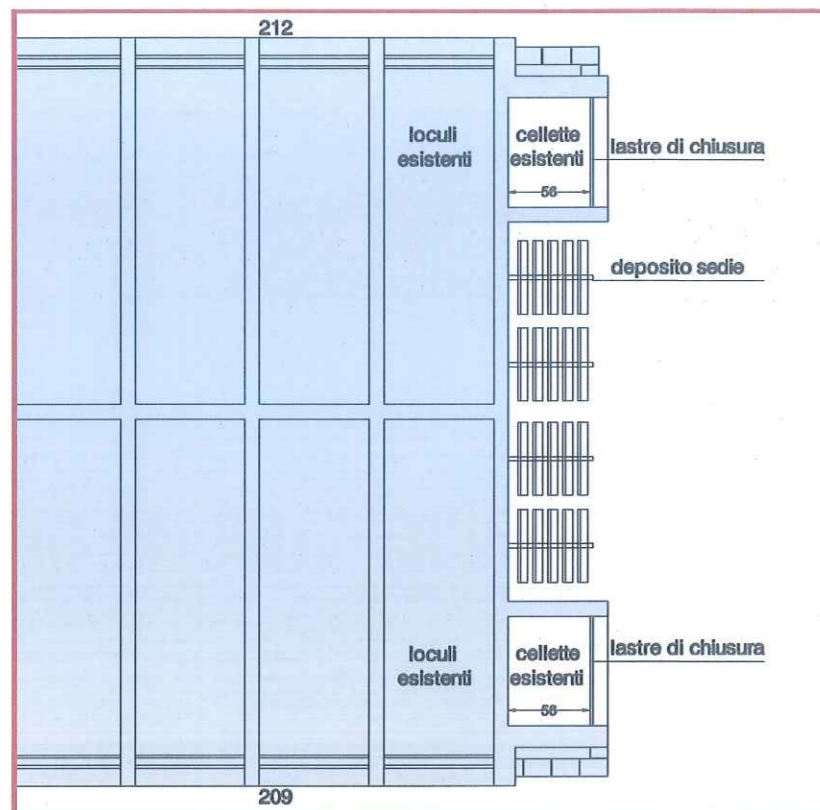
schema pianta scomparto tipo A - piano primo stato di fatto
