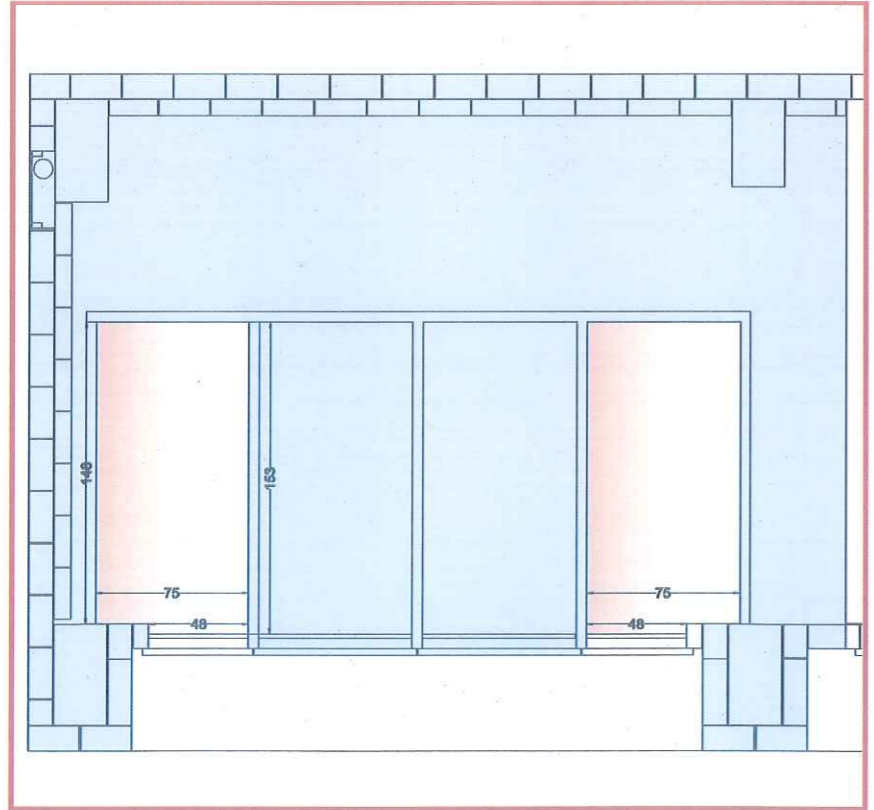
schema pianta scomparto tipo - cellari tipo 2 stato di fatto
