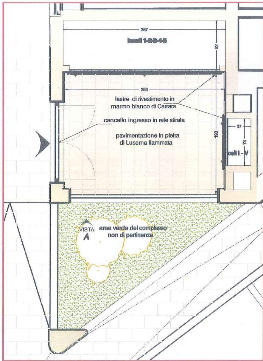
pianta TF1
