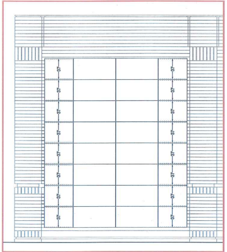
schema prospetto scomparto tipo - cellari tipo 2 stato di fatto
