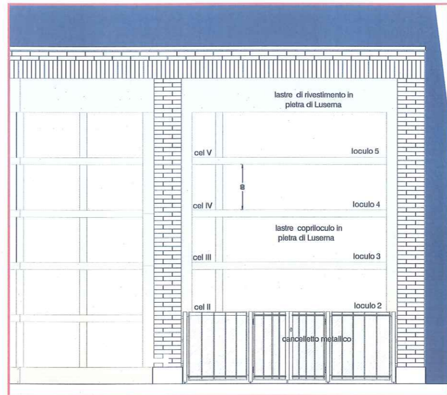
prospetto
