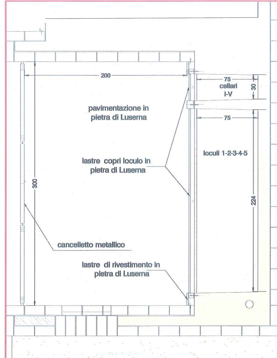
pianta TF tipo
