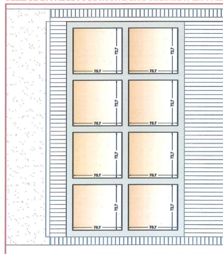
schema prospetto scomparto tipo B - piano terra stato di fatto
