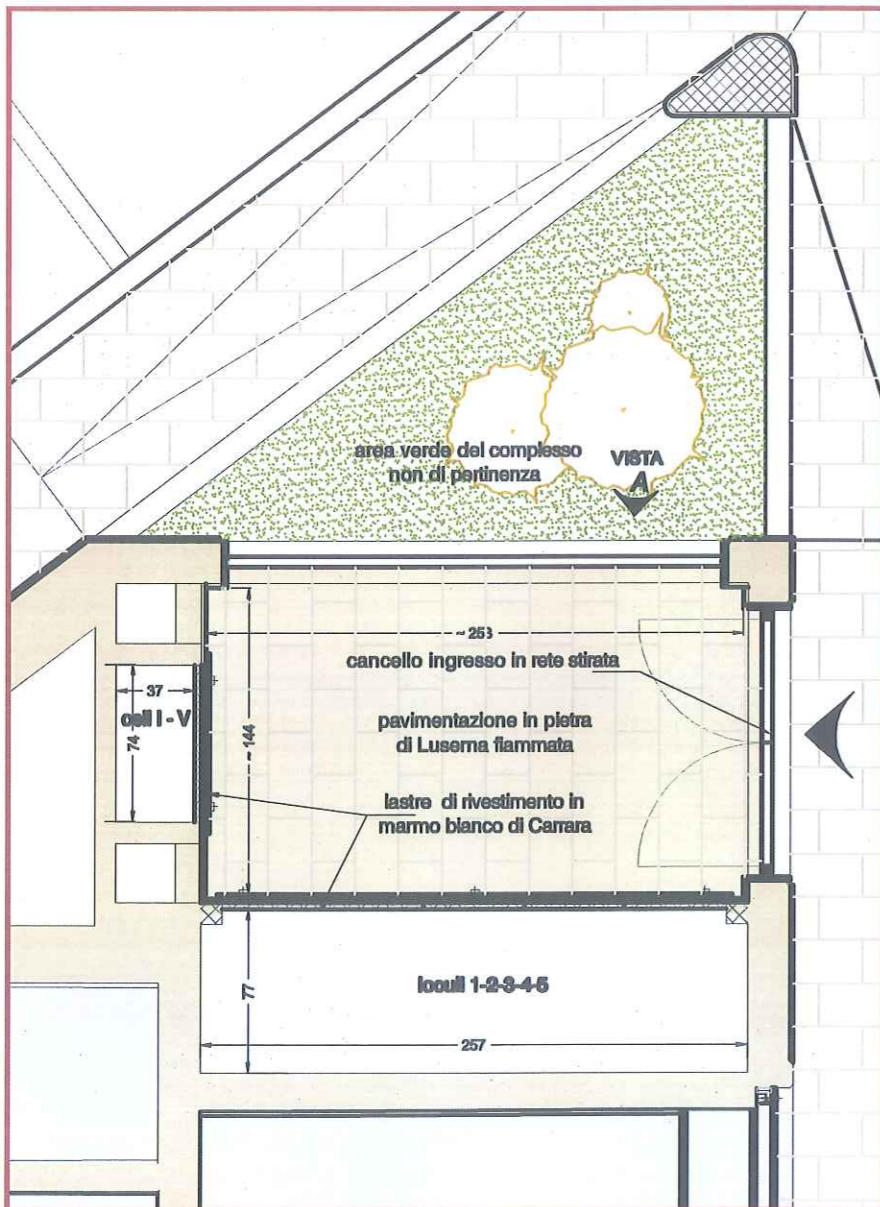
pianta TF8
