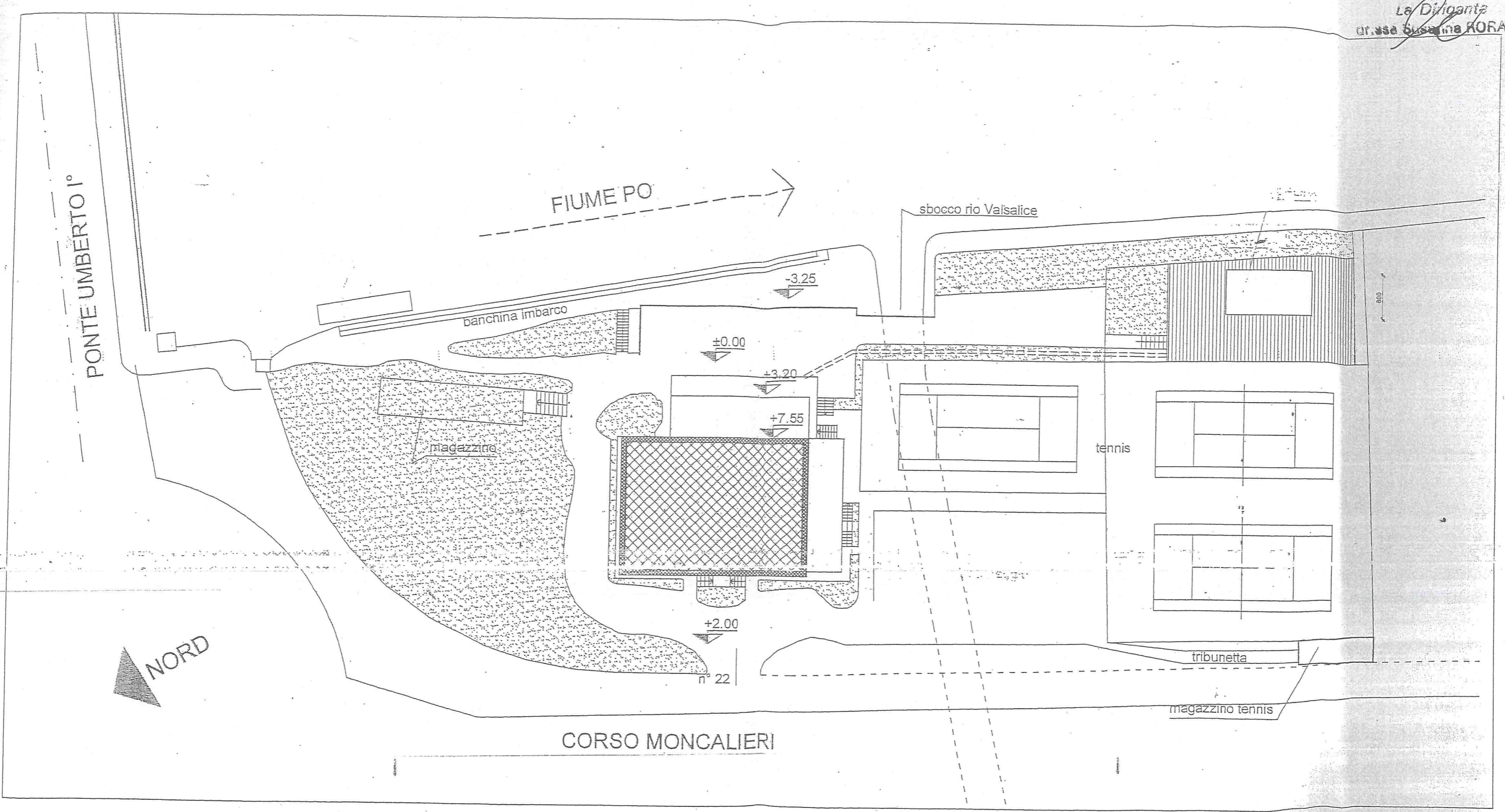
PLANIMETRIA - Scala 1:500 -
