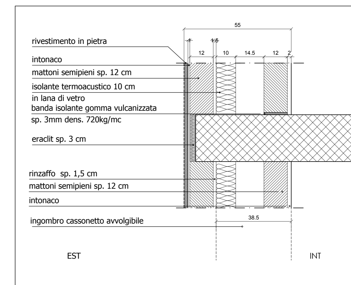
sezione tipo muratura perimetrale
