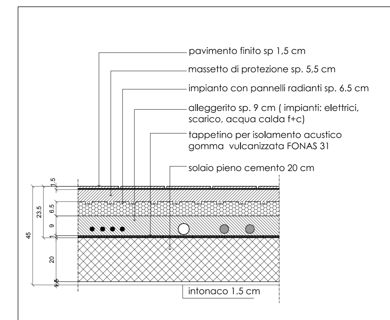
sezione tipo solaio interpianto
